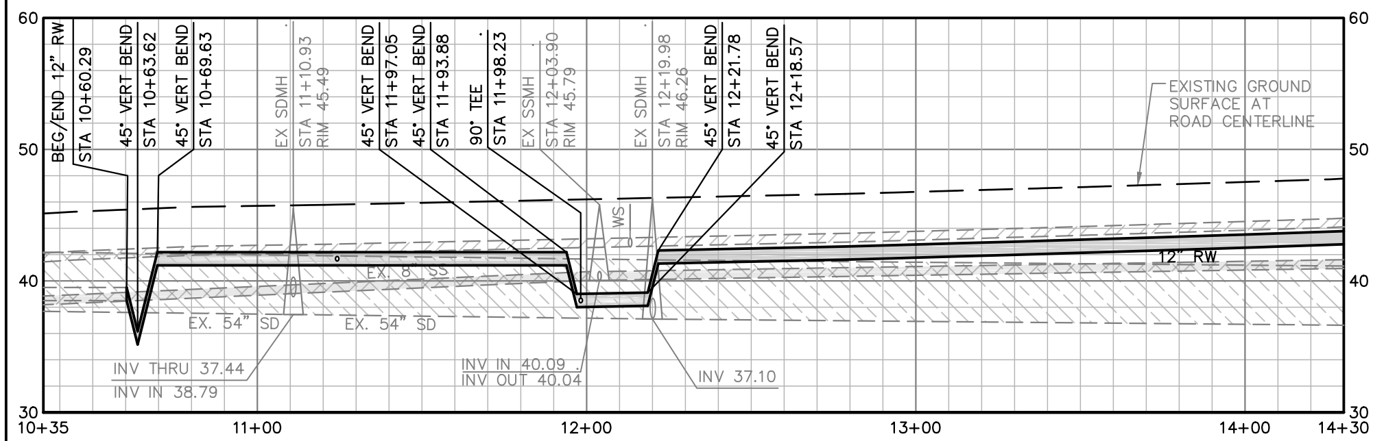
PROFILE STA 10+35 TO STA 14+30 SCALE: H: 1"=40'; V: 1"=10'
