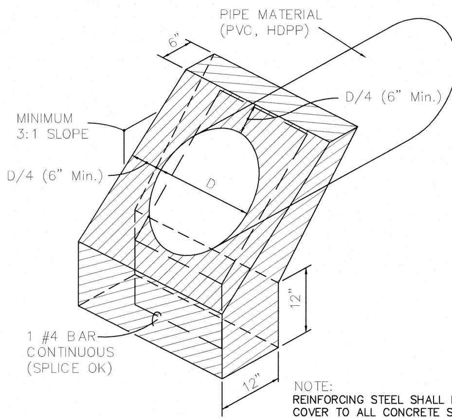
CONCRETE HEADWALL N.T.S.
