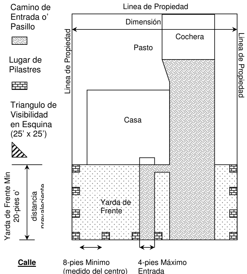
Ejemplo de Plan de Sitio Residencial- No ubicado en una Esquina
