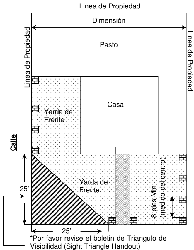
Ejemplo de Plan de Sitio Residencial- Lote de Esquina
