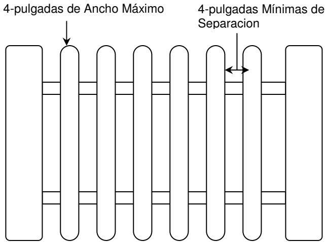
Ejemplo de Diseño de Cerca de Madera/Hierro Forjado
