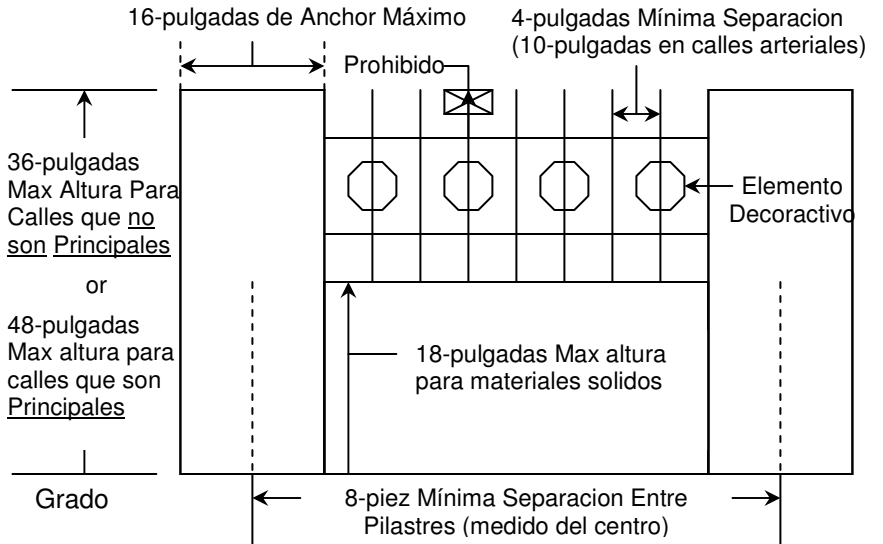
Ejemplo de Diseño de Cerca de Bloque o Ladrillo con Pilastres
