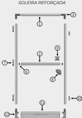
MOSQ. PORTA DE ABRIR SOLEIRA REFORÇADA
