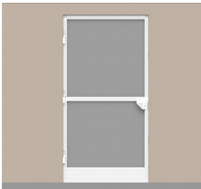
* INSTALAÇÃO DENTRO DO VÃO VISTA FRONTAL
