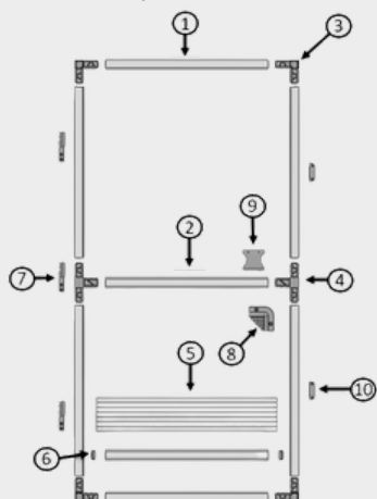
MOSQ. PORTA DE ABRIR
