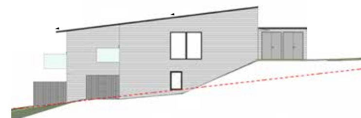
FASADER – VEST
