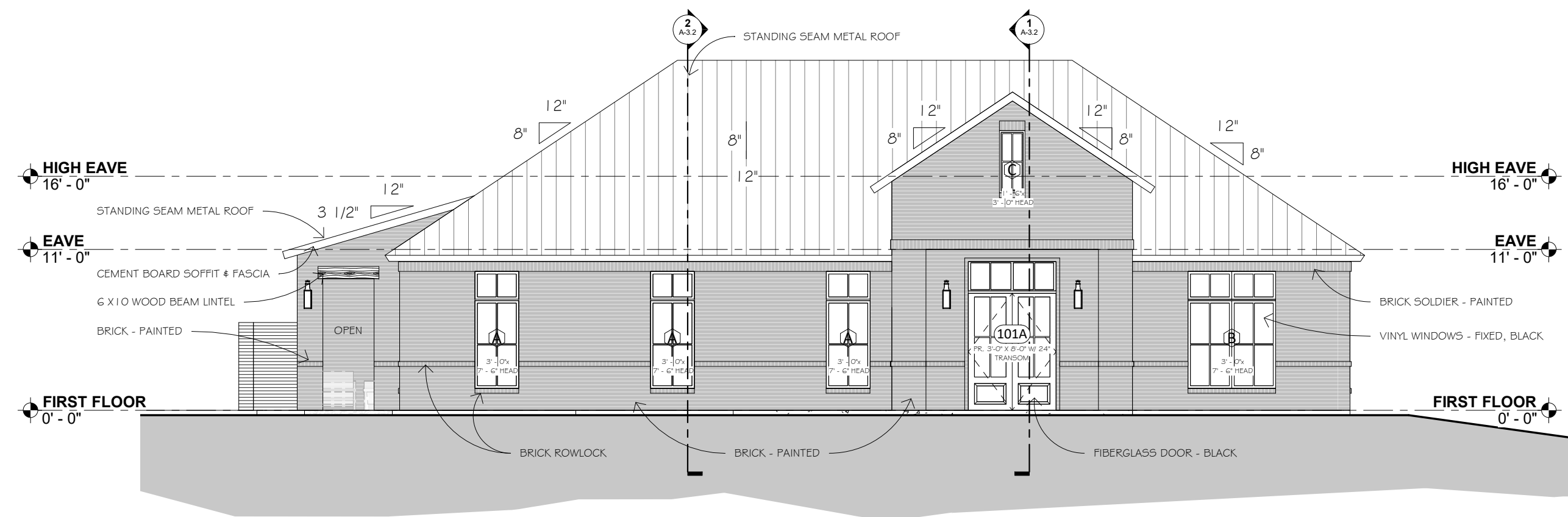
1 FRONT ELEVATION SCALE: 1/8" = 1'-0"
