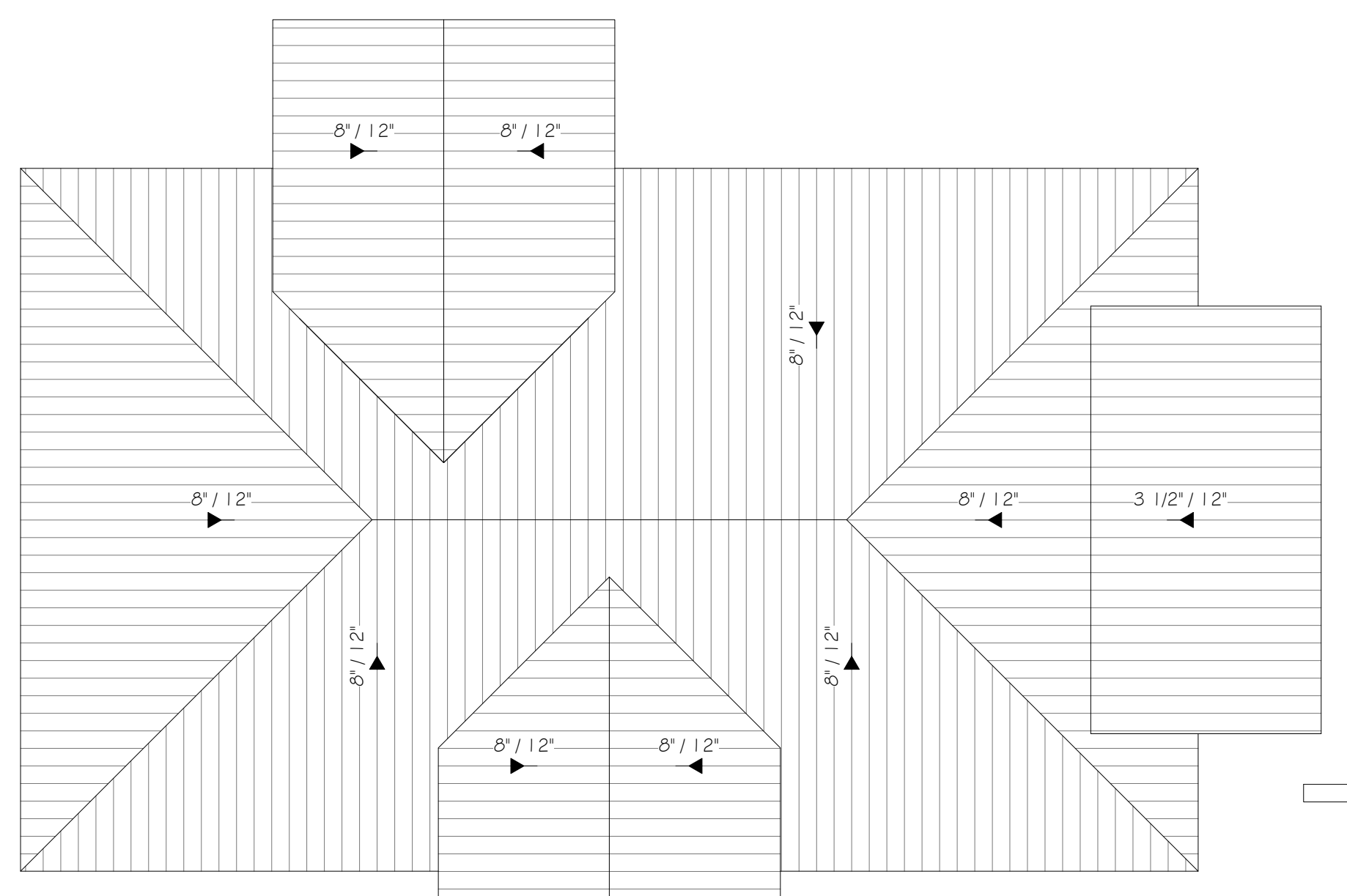
2 ROOF PLAN 1/8" = 1'-0" SCALE: 0'
