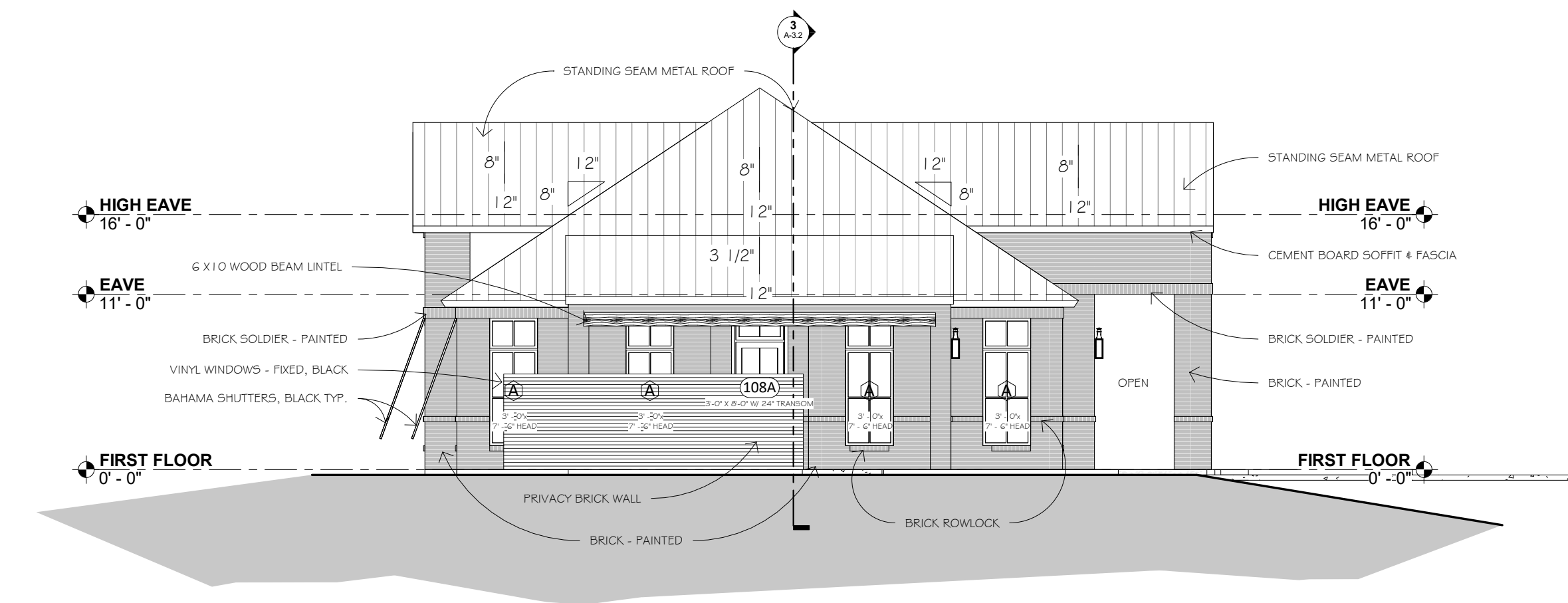
4 LEFT ELEVATION SCALE: 1/8" = 1'-0"
