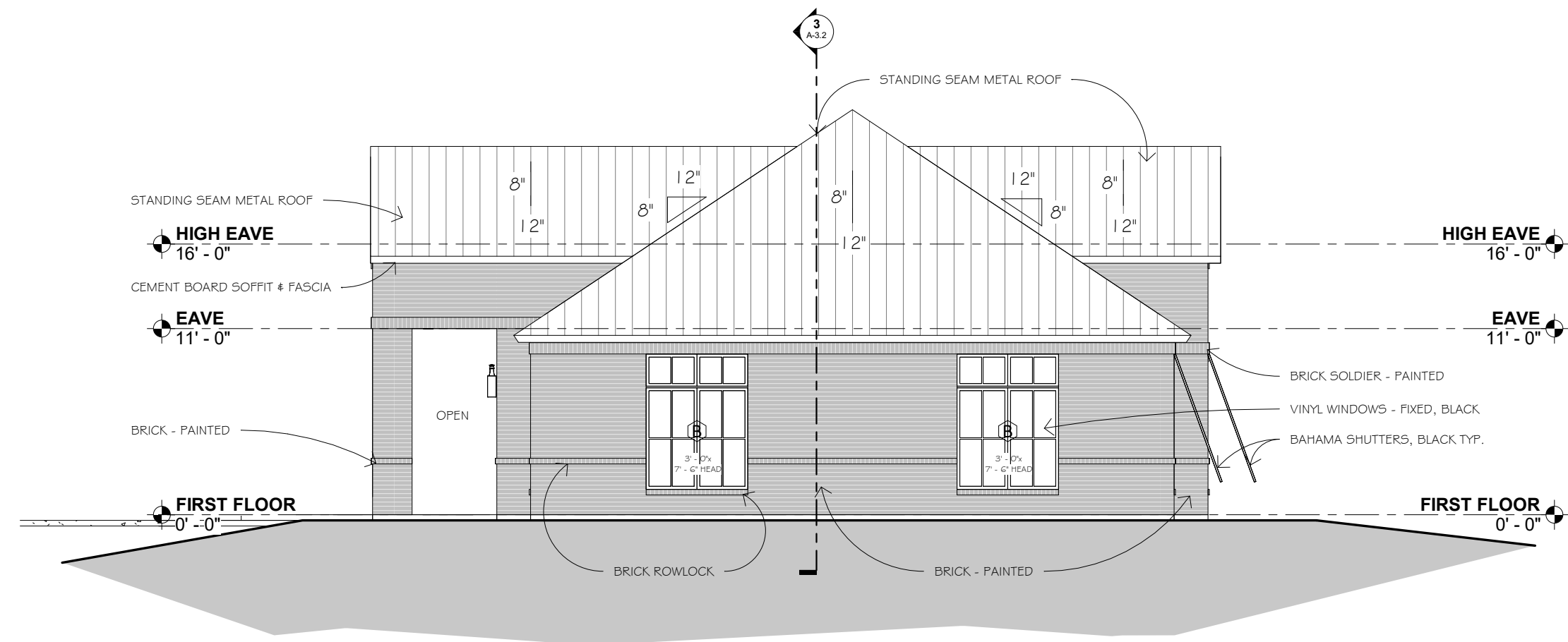
3 RIGHT ELEVATION SCALE: 1/8" = 1'-0"
