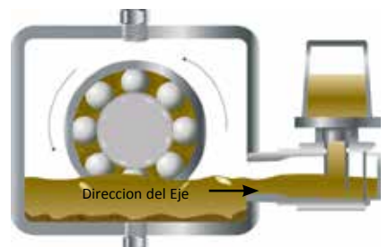
Aceitera de nivel constante instalada en la línea central del nivel deseado de aceite
