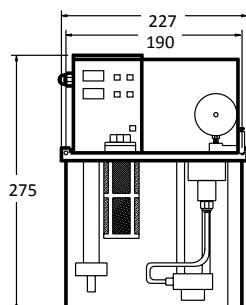
Depósito de 3 litros
