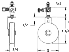
ENSAMBLAJE DE VÁLVULA Y ABRAZADERA GIRATORIA DISTANTE
