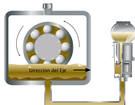
Aceitera de nivel constante despresurizada con conexión inferior
