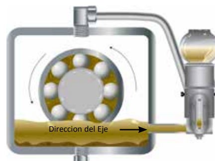
Aceitera de nivel constante con línea de balanceo de presión
