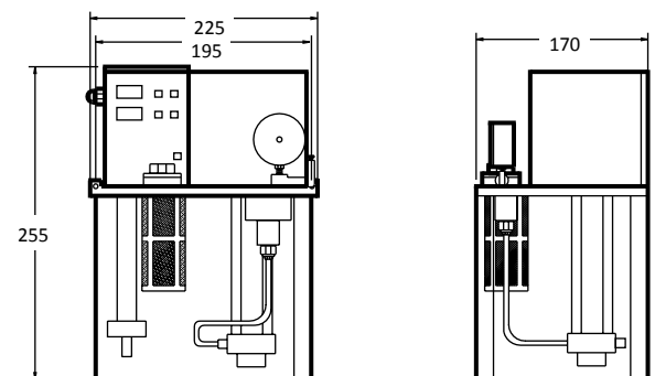
Depósito de 2 - 3 litros
