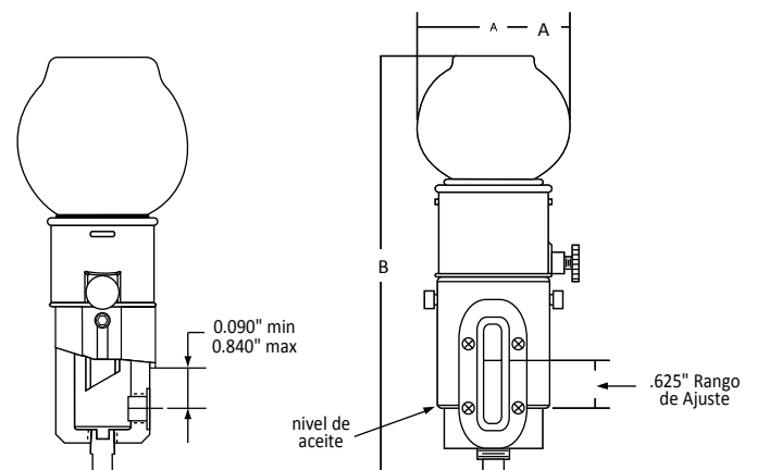
Aceitera Opto-Matic con línea de balanceo de presión
