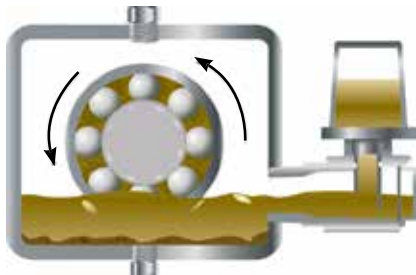
La Aceitera Watchdog® montada en línea divisoria central del nivel deseado de aceite
