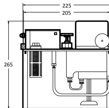
PE-40 y PE-50 Reservorios de 3 litros
