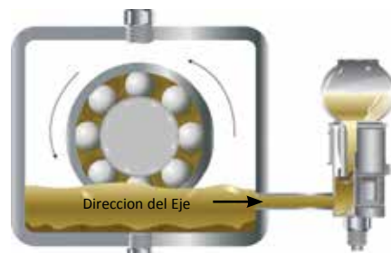
Aceitera de nivel constante despresurizada con conexión lateral
