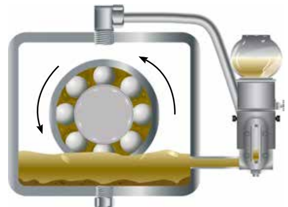
Aceitera Opto-Matic con línea de balanceo de presión
