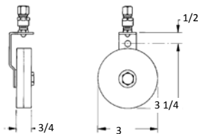
ABRAZADERA GIRATORIA DISTANTE PARA MANGUERA DE 1/4"
