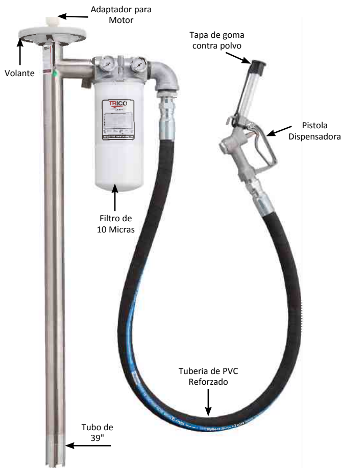
Sistema de filtración para Barriles – P/N 30035
