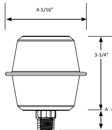
Cámara de expansión a temperatura alta
