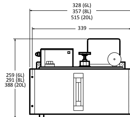
PE-40 y PE-50 Reservorios de 6, 8, y 20 litros (Nota: Todas las dimensiones son en mm.)
