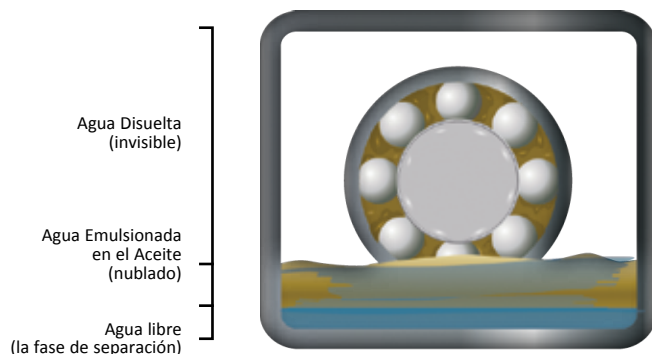
Tres etapas de agua dentro de un aceite lubricante.
