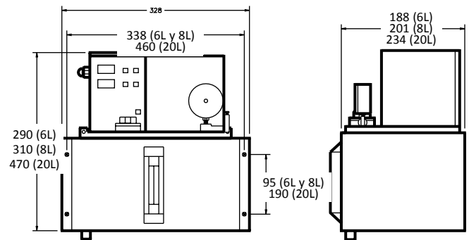
Depósitos de 1 - 6, 8 y 20 litros
