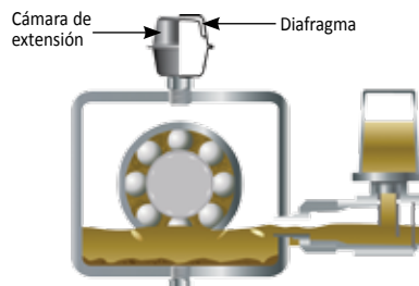
Cámara de expansión a temperatura alta
