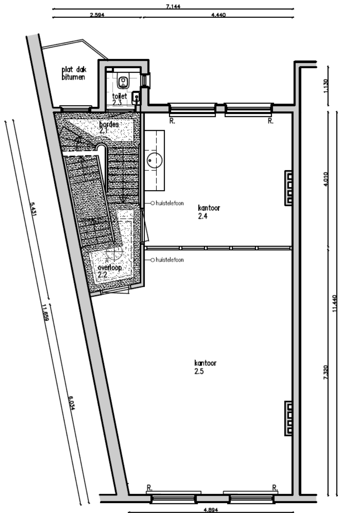
2e VERDIEPING
