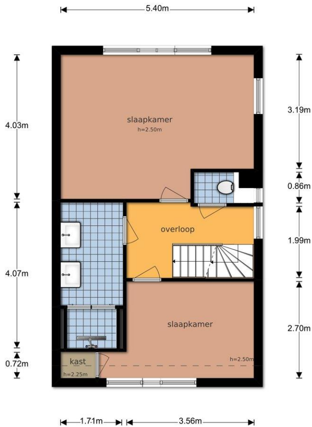
Van Den Bergstraat 14 - Oud-Beijerland Eerste Verdieping
