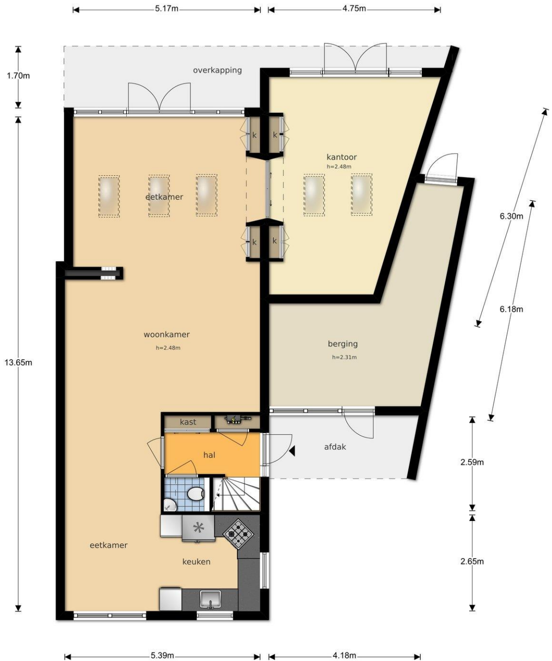
Van Den Bergstraat 14 - Oud-Beijerland Begane Grond
