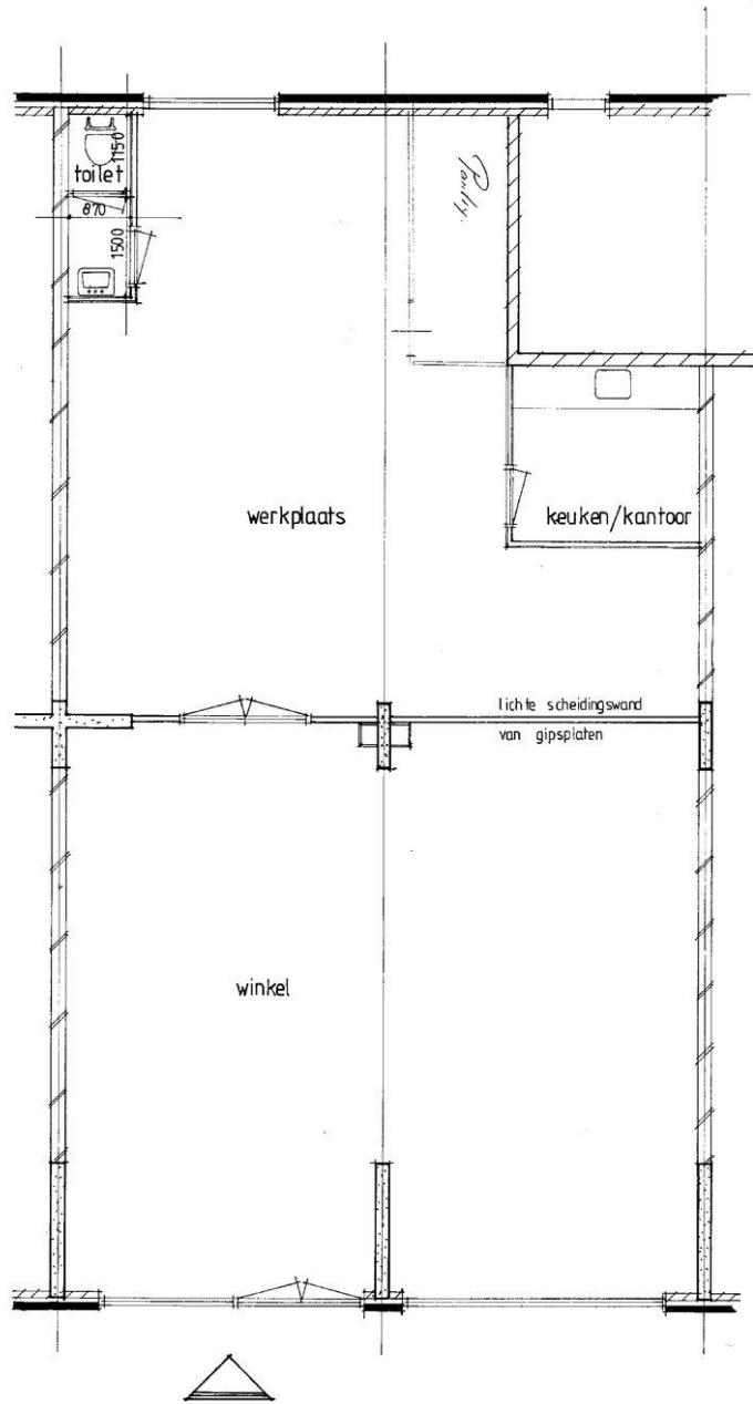
Plattegrond RIJWELHANDEL STEVE BIKOLAAN 193_195
