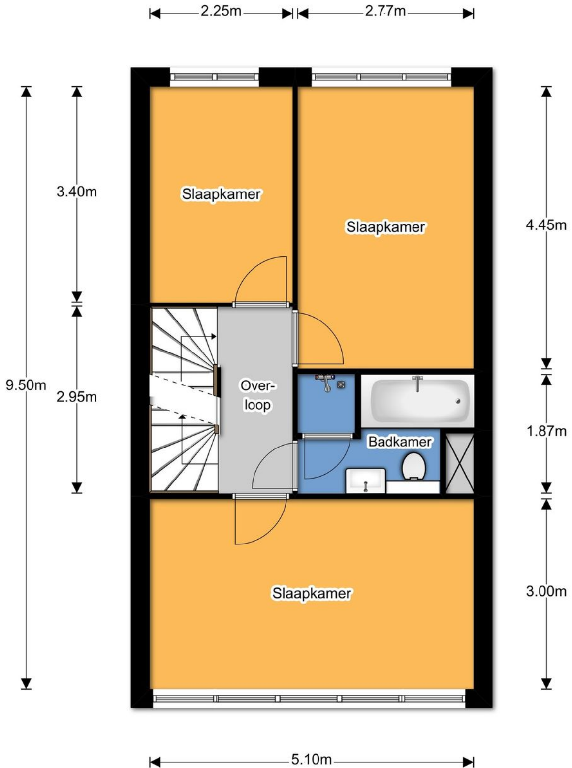
1e verdieping
