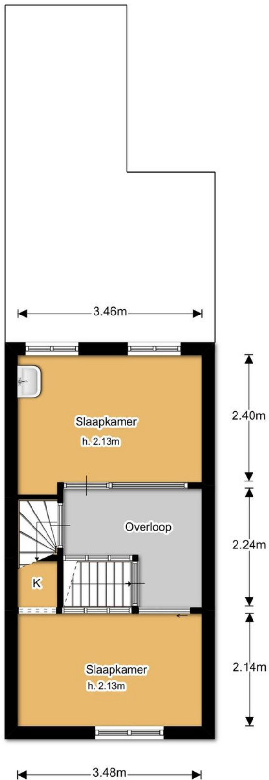
Eerste verdieping
