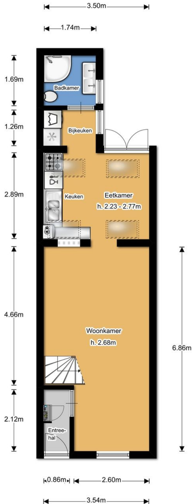
Begane grond
