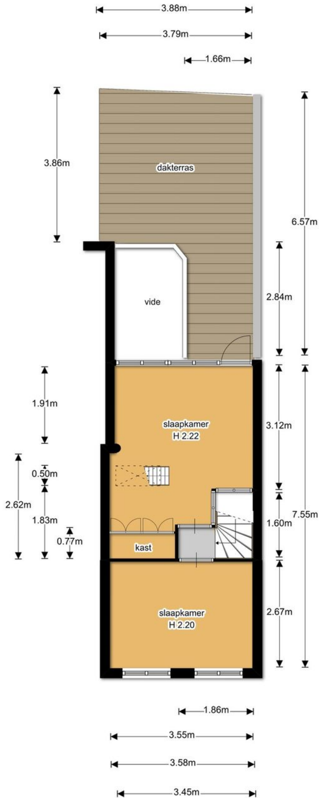
eerste verdieping
