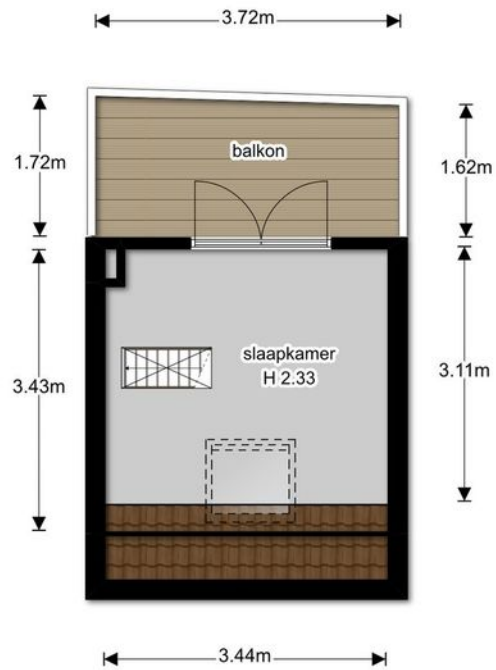
tweede verdieping
