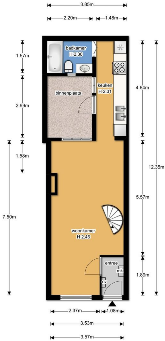
begane grond
