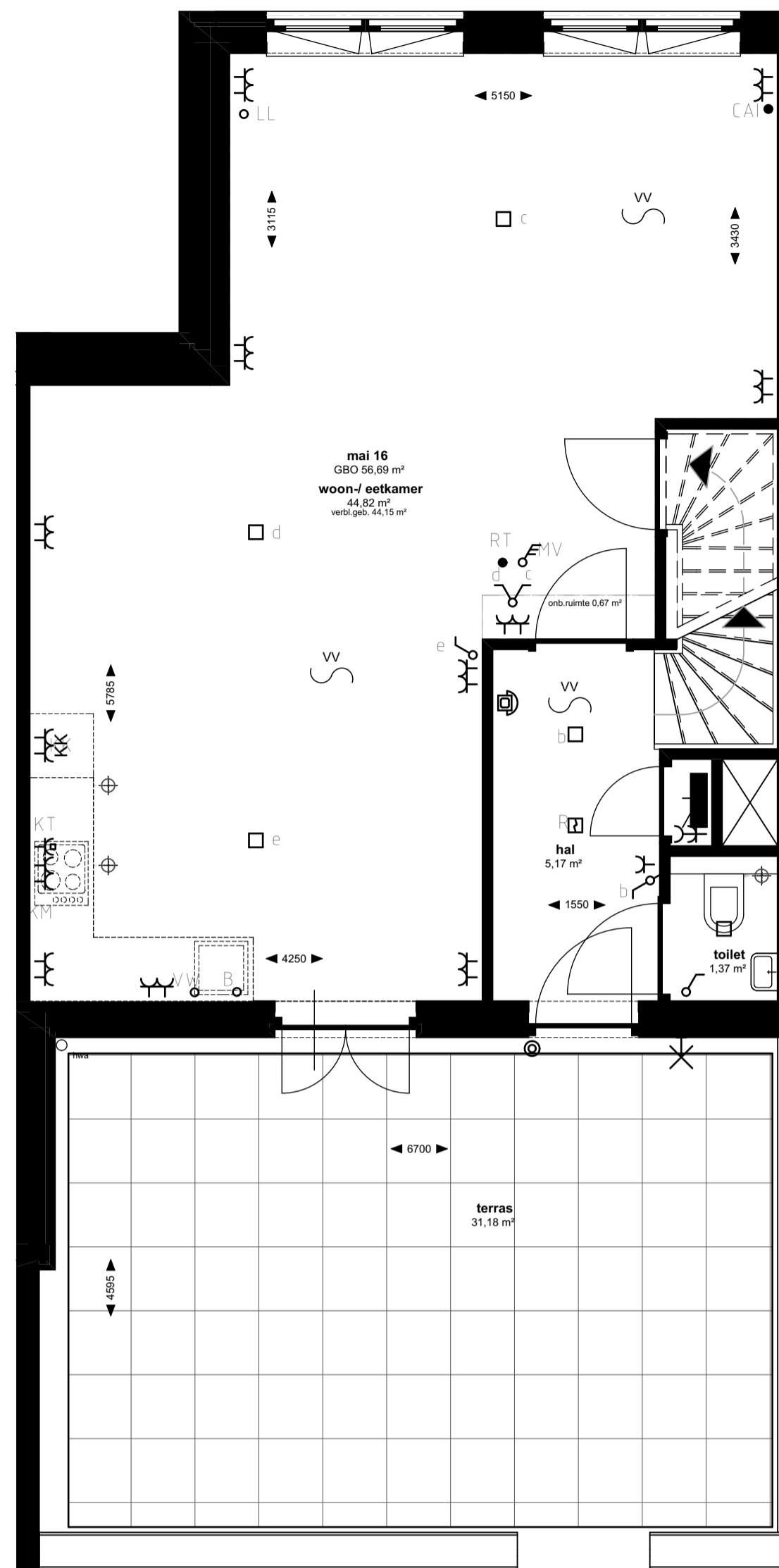
Maisonnette 16 - niveau 1 (1:50)
