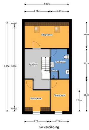
2e verdieping
