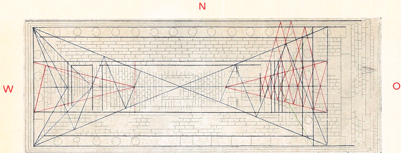
Fig. 10. Grundrißkonstruktion des Tempels C
