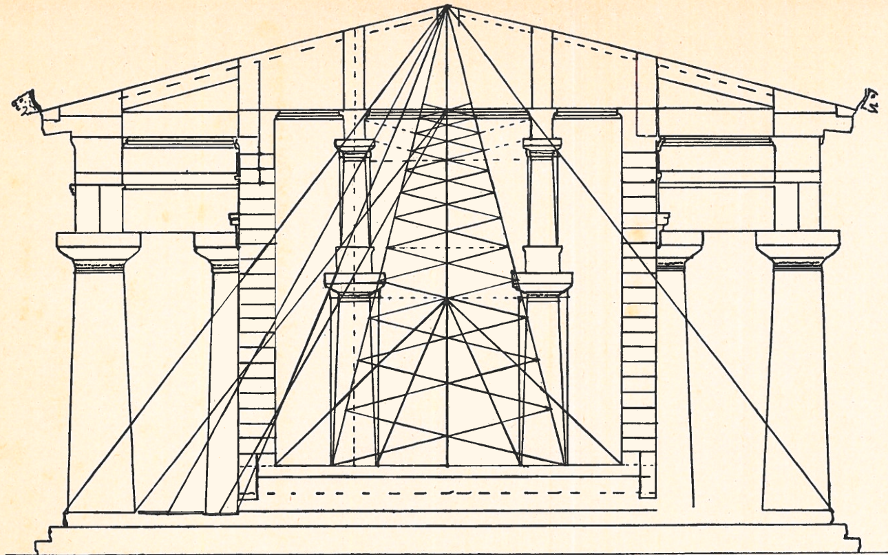
Fig. 2. Querschnitt durch den Poseidontempel zu Paestum
