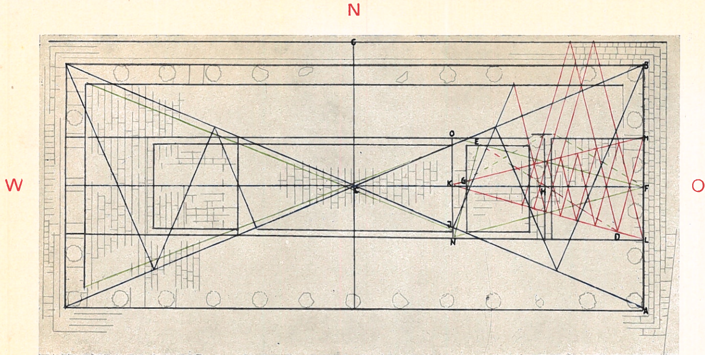
Fig. 8. Grundrißkonstruktion des Tempels D
