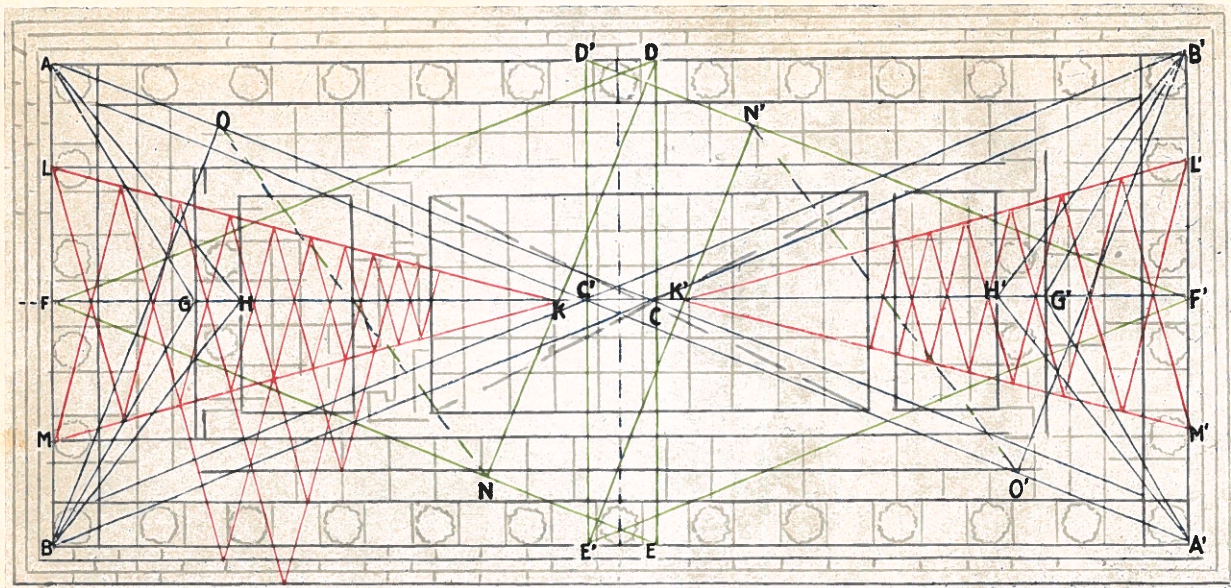
Fig. 9. Grundrißkonstruktion des Concordiatempels
