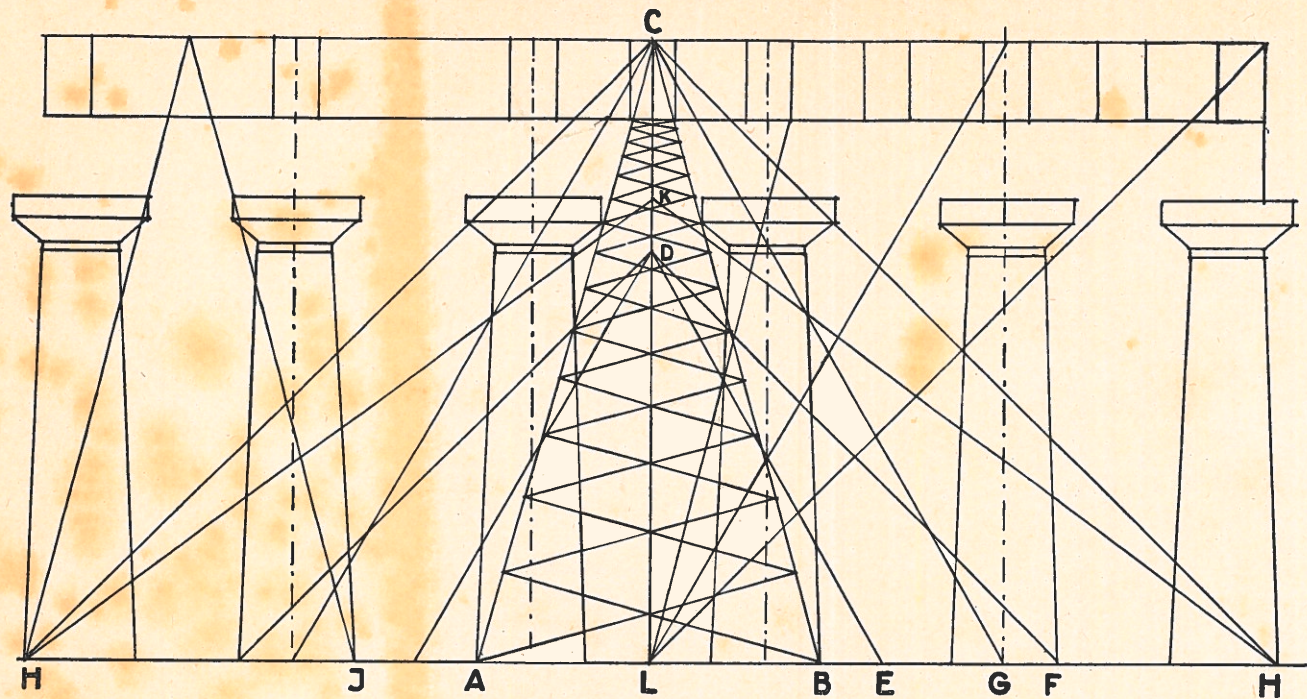
Fig.1. Front des Poseidontempels zu Paestum
