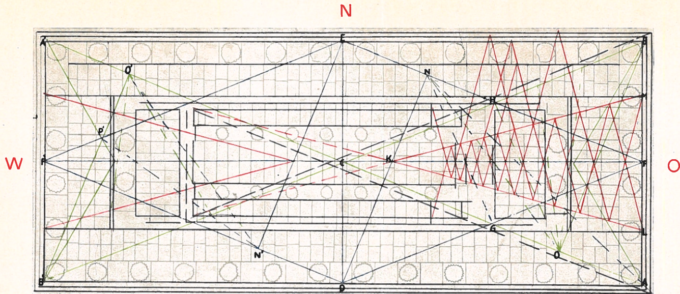
Fig. 7. Grundrißkonstruktion des Poseidontempels
