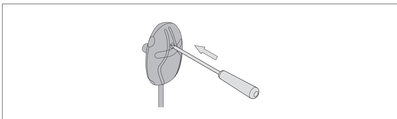
Figure 10. Reset button of the overheat protector Figure 10. Bouton de réinitialisation de la sécurité-surchauffe
