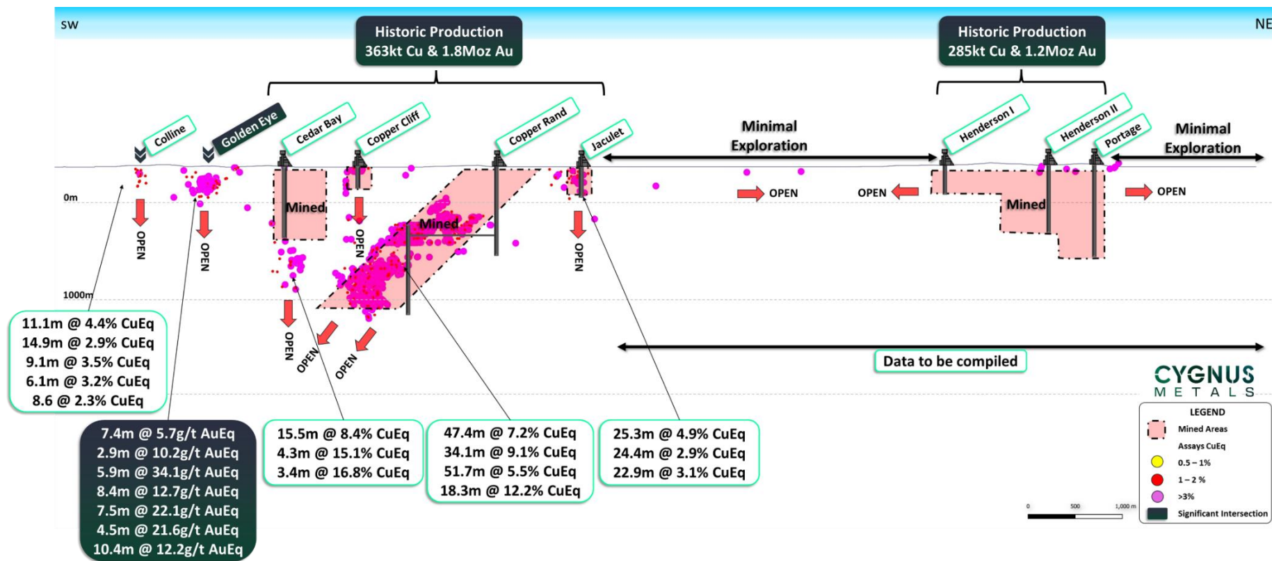
Figure 2 : Section longitudinale composite traversant le camp de Chibougamau Nord illustrant Golden Eye avec des intersections allant jusqu'à 5,9 m @ 34,1 g/t ÉqAu. Se référer aux communiqués de la TSXV/ASX datés du 15 octobre 2024 et du 24/25 mars 2025 pour les résultats de forage annoncés antérieurement.
