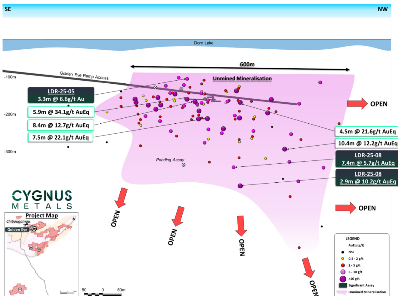
Figure 1 : Section longitudinale composite de Golden Eye sur 600 m de longueur avec des teneurs en or significatives allant jusqu'à 34,1 g/t ÉqAu sur 5,9 m. La minéralisation reste ouverte en profondeur avec 2,9 m @ 10,2 g/t ÉqAu recoupée dans le sondage LDR-25-08. Se référer à l'annexe A du présent communiqué pour les nouvelles intersections de forage et aux communiqués de la TSXV/ASX datés du 15 octobre 2024, du 24/25 mars 2025 et du 16/17 avril 2025 pour les résultats de forage annoncés antérieurement.
