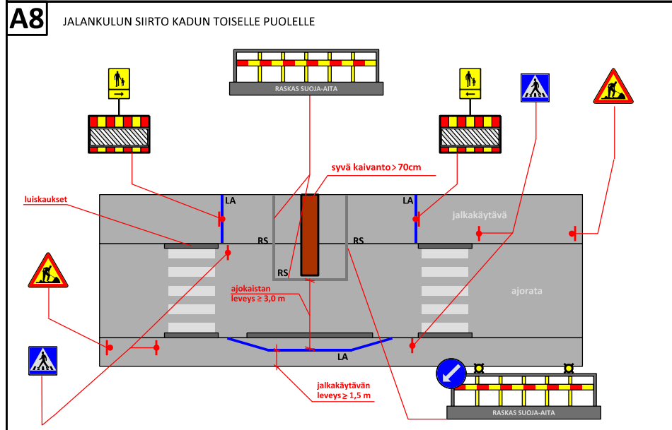
LIIKENNEJÄRJESTELYIDEN TYYPPIKUVAT A7 - 8 Kaivutyöt, tonttiliittymät; Ei kaivuaikainen tilanne
