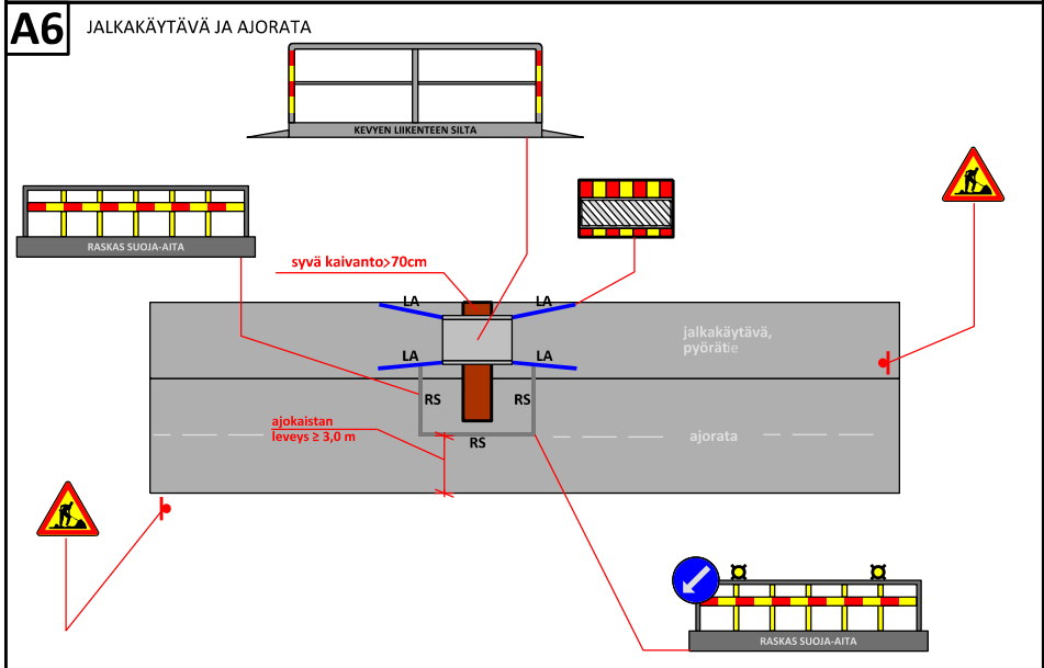
LIIKENNEJÄRJESTELYIDEN TYYPPIKUVAT A5 - 6 Kaivutyöt, tonttiliittymät; Ei kaivuaikainen tilanne
