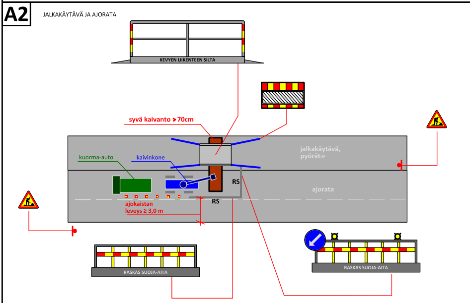
LIIKENNEJÄRJESTELYIDEN TYYPPIKUVAT A 1 - 2 Kaivutyöt, tonttiliittymät; Kalvuakalnen tilanne
