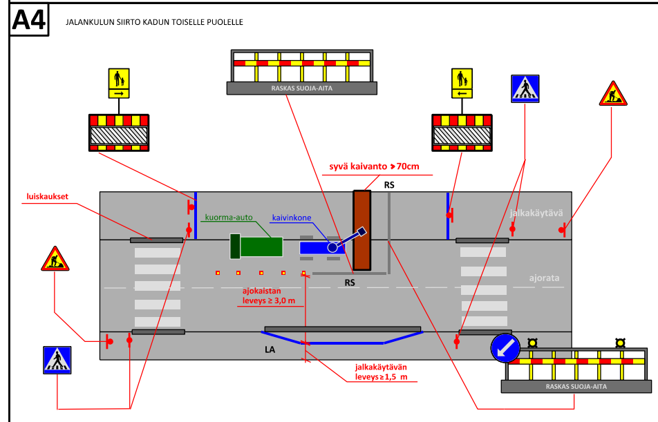
LIIKENNEJÄRJESTELYIDEN TYYPPIKUVAT A 3 - 4 Kaivutyöt, tonttiliittymät; Kaivuaikainen tilanne
