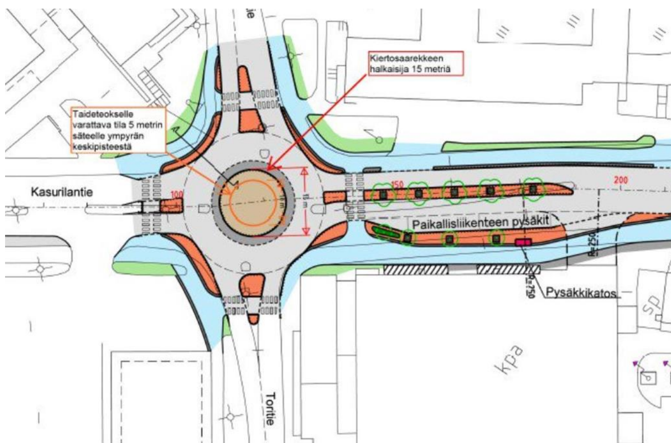
Kuva 2. Kasurilantien kiertoliittymä.
