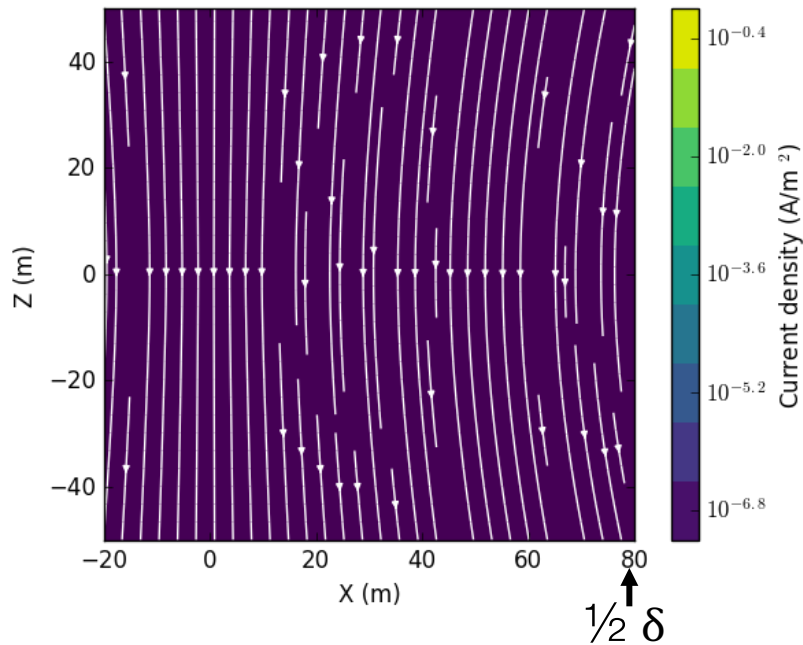
EM induction
