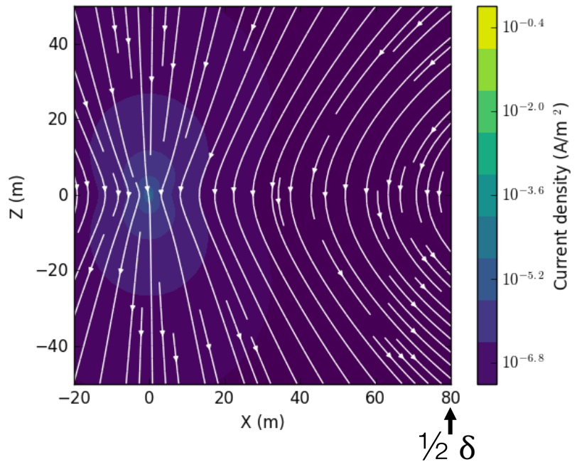
EM induction
