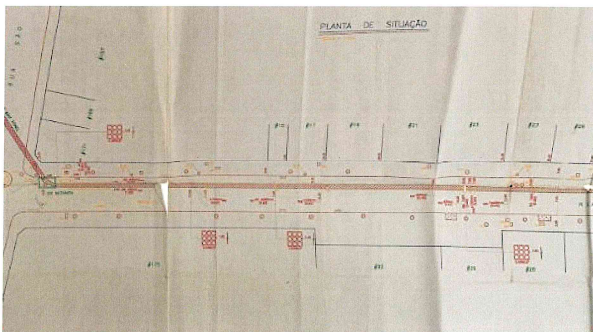
Figura 06 – Rua Barão de Lucena com a Rua São Clemente (redes de alta tensão)
