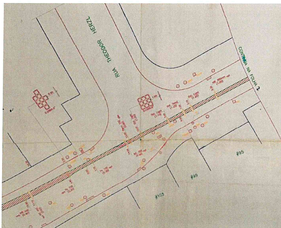
Figura 04 – Rua Barão de Lucena com a Rua Theodor Herzl (redes de alta tensão)
