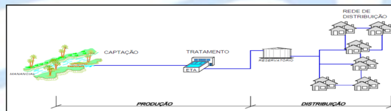
FIGURA 1 – ESQUEMA SIMPLIFICADO DE UM SISTEMA DE ABASTECIMENTO
