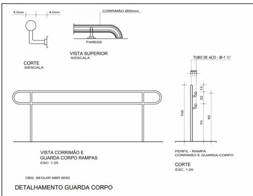
Figura 36 - Acessibilidade das rampas e acessos internos do empreendimento
