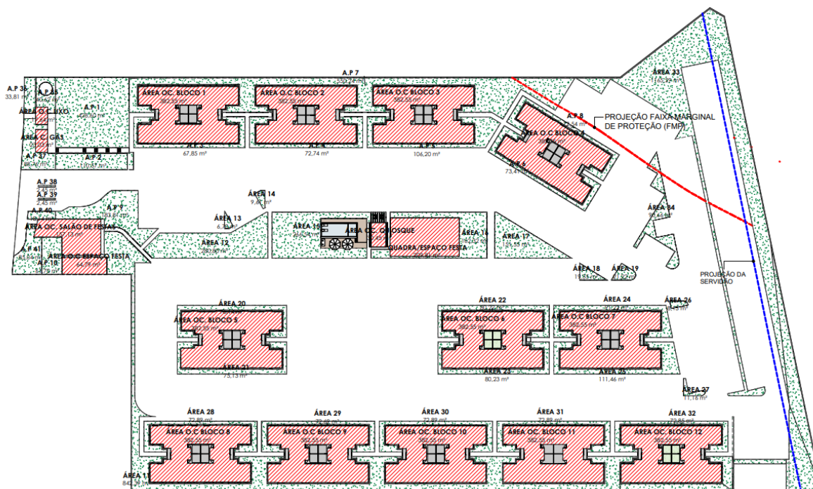
PLANTA DE ÁREAS PERMEÁVEIS E TAXA DE OCUPAÇÃO
