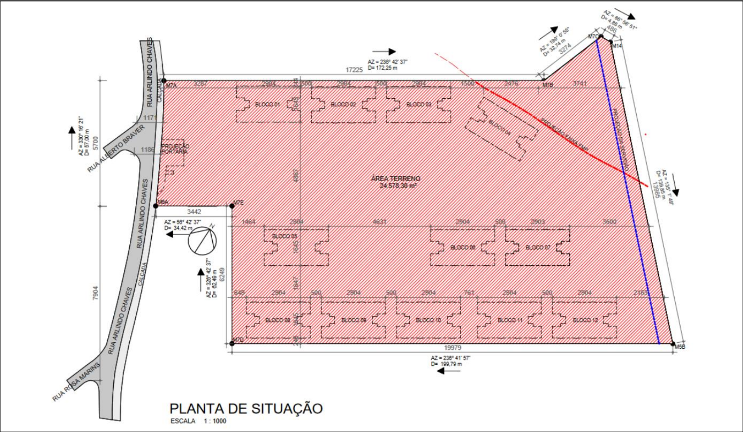
MAPA 02 - PLANTA DE SITUAÇÃO
