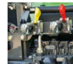
Le freinage pneumatique à deux lignes agit également sur la remorque quand le frein de stationnement est activé.
