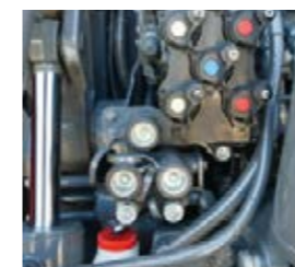
Les raccords hydrauliques sont marqués de différentes couleurs. Vous pouvez ainsi raccorder vos outils rapidement et en toute sécurité.
