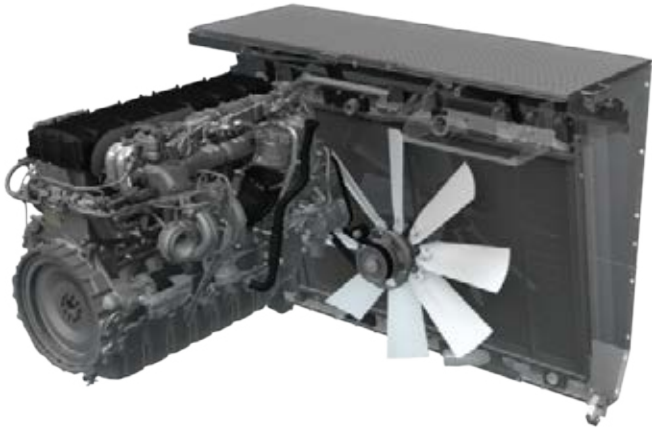
Het koeloppervlak bedraagt 2,7 m² en hoeft dankzij AirSense® Cooling binnen het seizoen niet handmatig te worden gereinigd.
