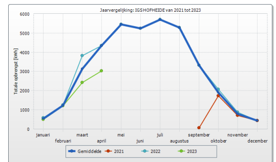
Opbrengst zonnepanelen
