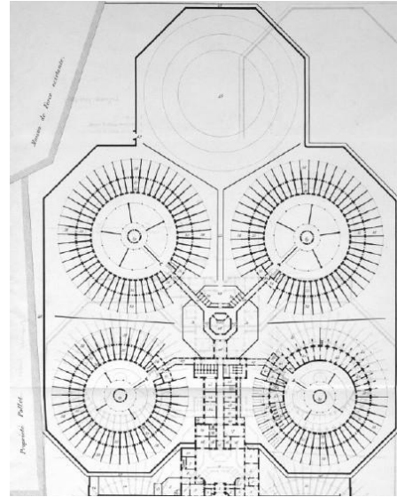
Figuur 3: Koepelmodel van Derré (Foto van het boek: PENITENTIAIRE INRICHTING DE NIEUWE-WANDELING GENT. (Ed.). (2011). 150 jaar Nieuwewandeling. Gevangenis Gent, 1862 - 2012. Gent Uitgeverij Snoeck, pagina 57
