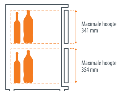
Ladesegment E3/3DA
