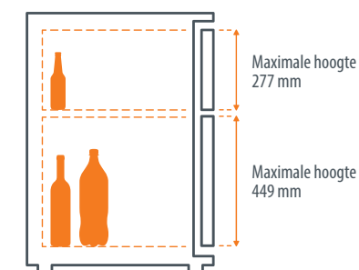
Ladesegment E3/5DA
