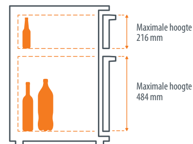
Ladesegment X/7DA
