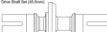
OD2415 リジッドアクスル(For GALM/スチール) Rear Spool Axle (For GALM/Steel)
