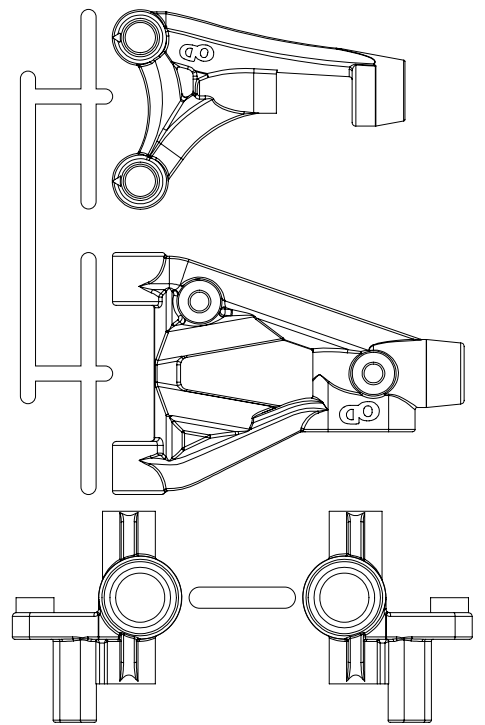
OD2257 フロントサスアーム&ナックルセット (For XEX spec.R, OD) Front Suspension Arm & Knuckle Set (For XEX spec.R, OD)
