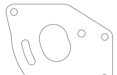
OD2414 モータープレート (For GALM/ブラック) Motor Plate (For GALM/Black)
