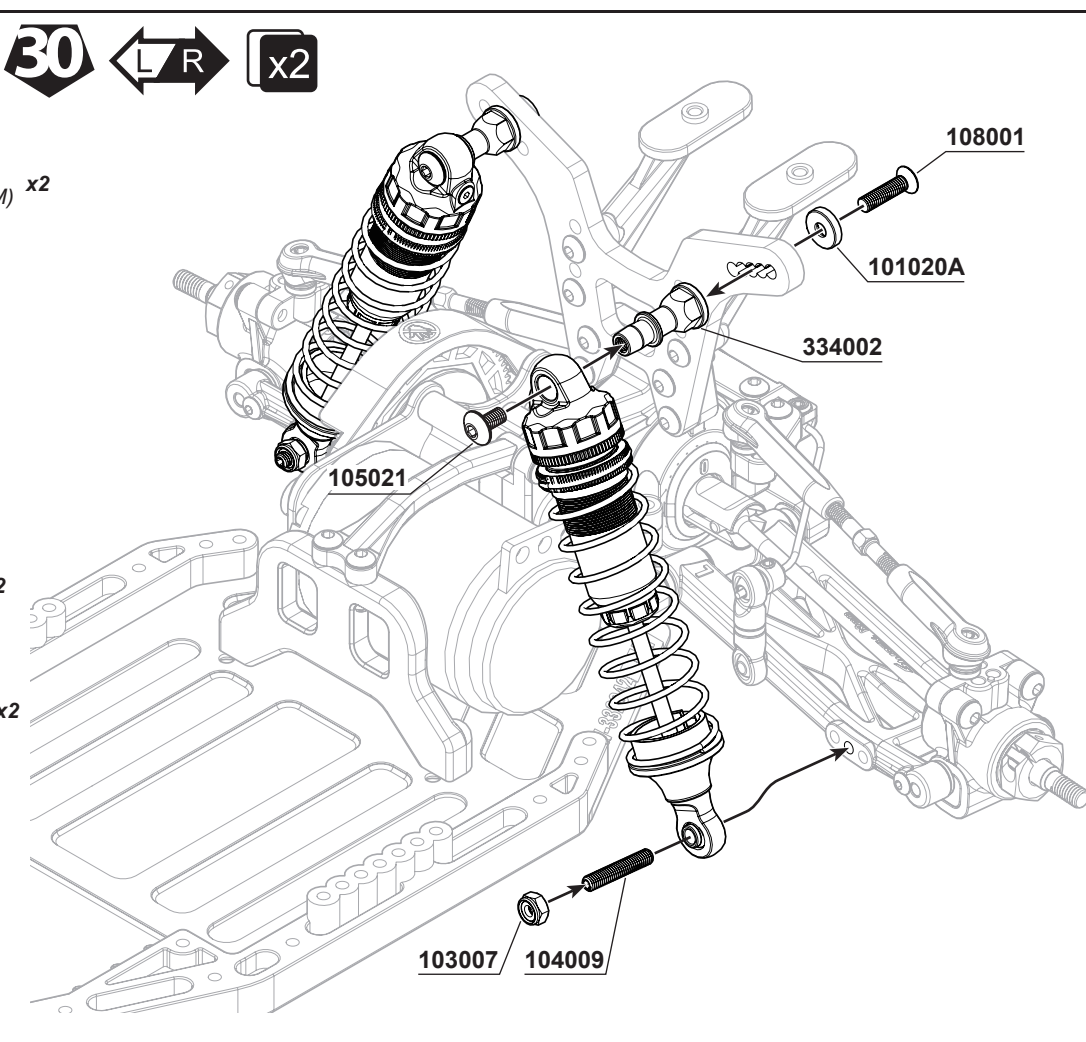
334002 Aluminum Shock Cap Stud x2
