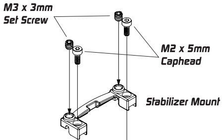
Stabilizer Mount XP-10230
