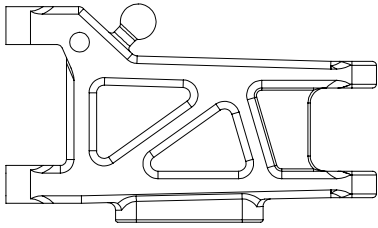
Composite Suspension Arm Rear XP-10276 Optional XP-10459
