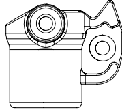
Composite Steering Block Left XP-10277 Optional XP-10462 , XP-10389
