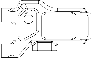
Composite Suspension Arm Front XP-10276 Optional XP-10459
