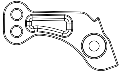
Composite Steering Block Plate Right XP-10109 Optional XP-10247
