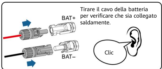
Terminali batteria (BAT+/BAT-)
