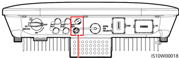
Terminali batteria (BAT+/BAT-)
