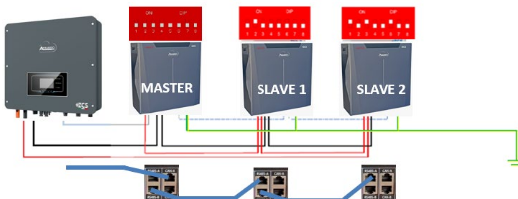
Figura 61 – Collegamento in parallelo con 5K3XP Master e 5K3 Slave
