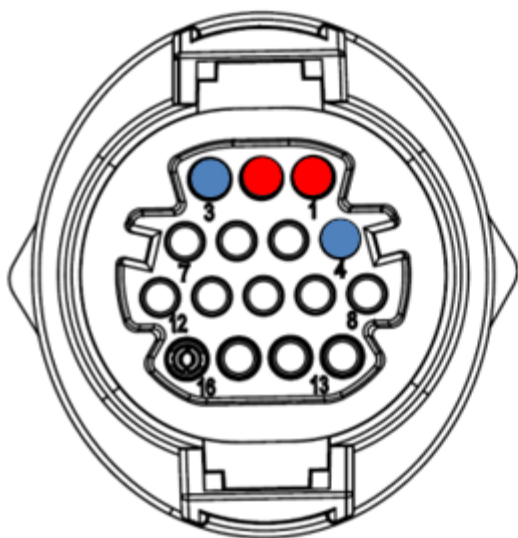
Figura 146 – Collegamento della linea seriale tramite connettore di comunicazione per 3PH HYD5000-HYD20000-ZSS
