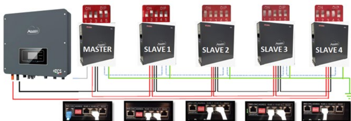
Figura 28 – Collegamento in parallelo di cinque batterie WeCo 4k4
