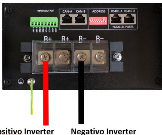
Figura 31- Collegamento del cavo di potenza dalla batteria Weco 4k4 PRO all'inverter
