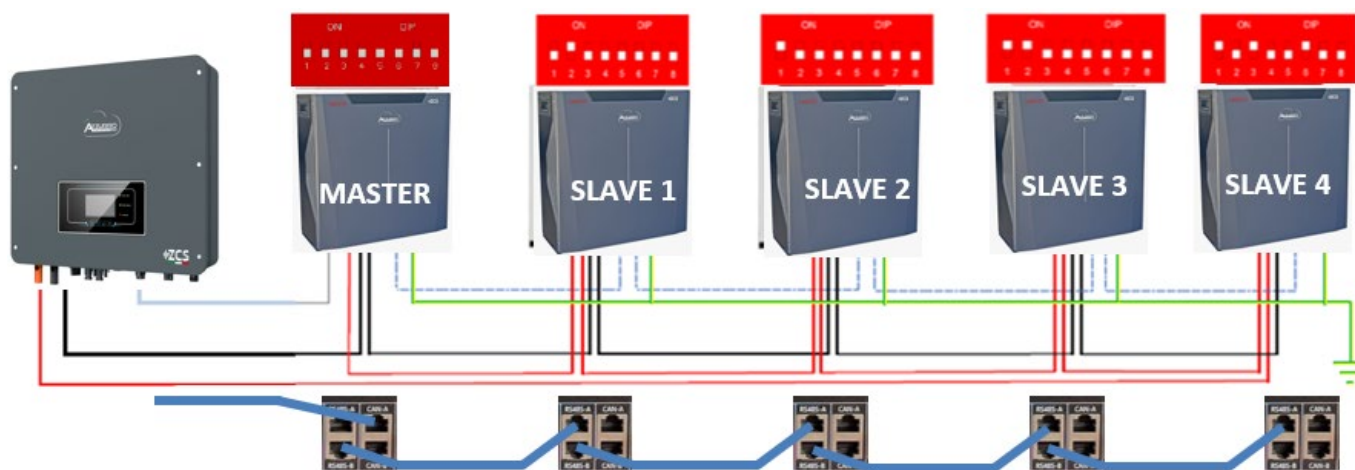
Figura 63 – Collegamento in parallelo con 5K3XP Master e 5K3 Slave
