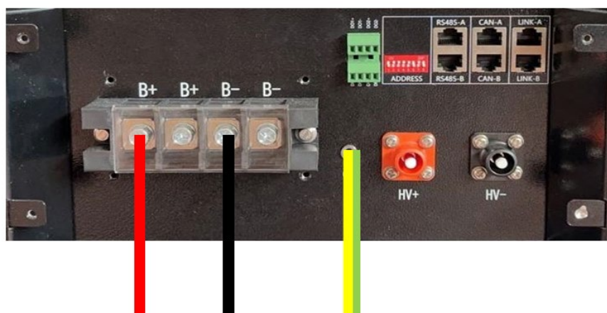
Figura 54 – Collegamento della batteria WeCo 5K3XP
