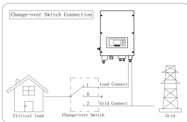
Figura 6 – Collegamento del commutatore
