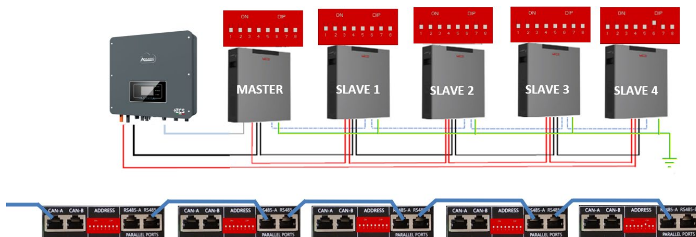
Figura 44 – Collegamento in parallelo di cinque batterie WeCo 4k4-LT
