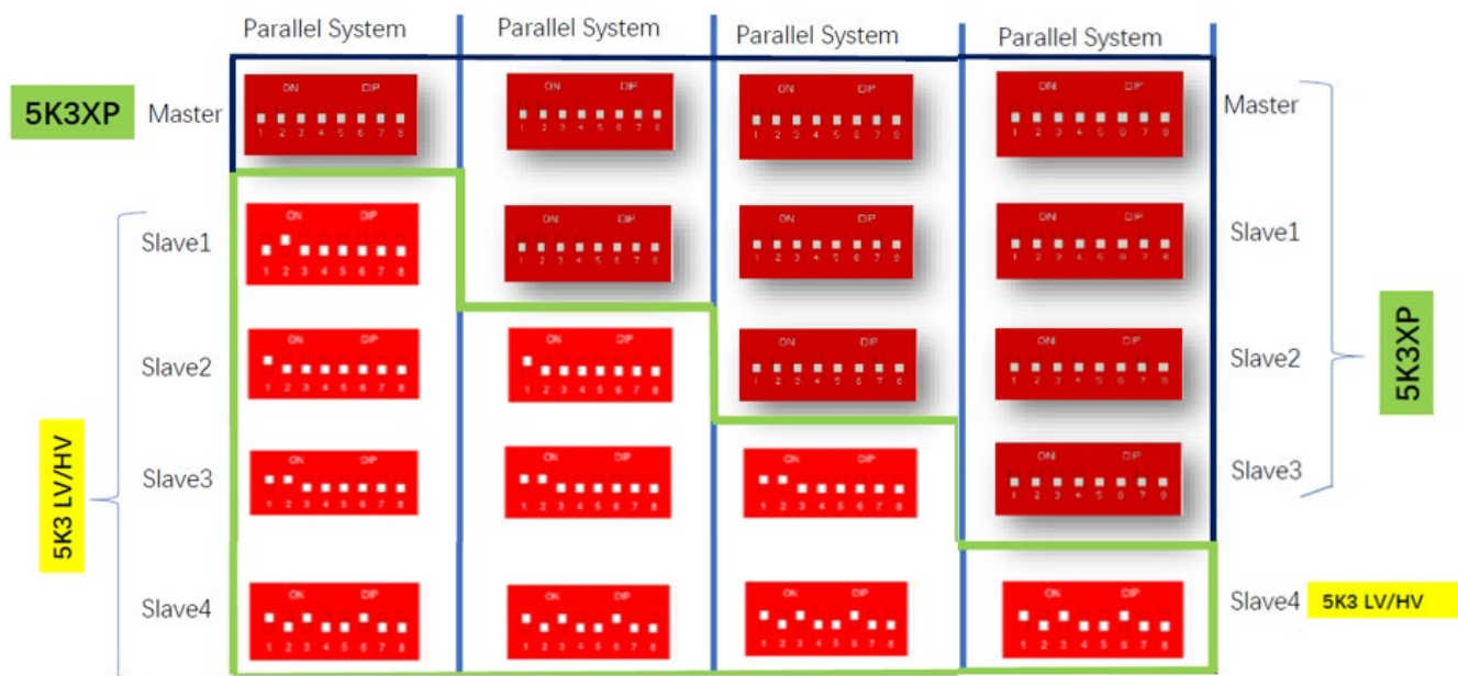
Figura 60 – Collegamento in parallelo di batterie WeCo 5K3XP e WeCo 5K3
