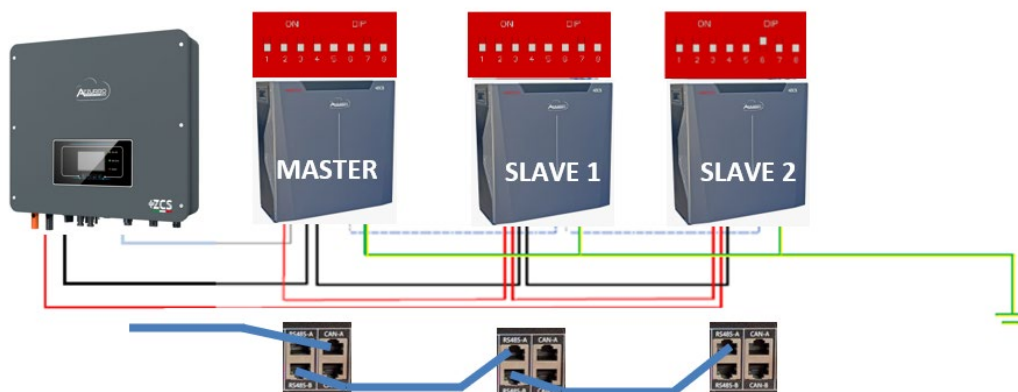
Figura 57 – Collegamento in parallelo di tre batterie WeCo 5K3XP
