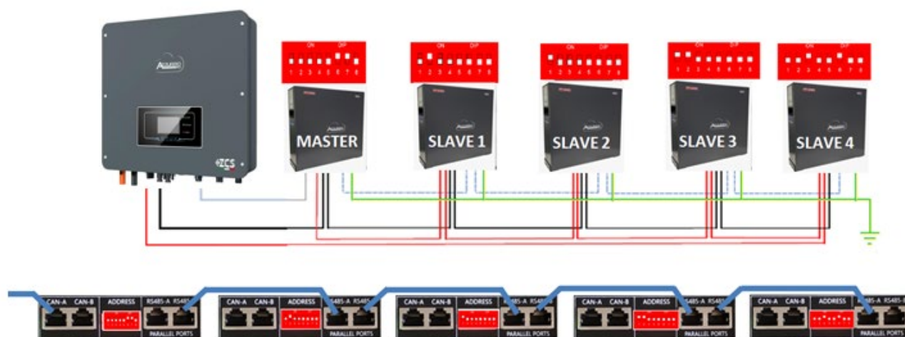
Figura 36 - Collegamento in parallelo di cinque batterie WeCo 4k4 PRO
