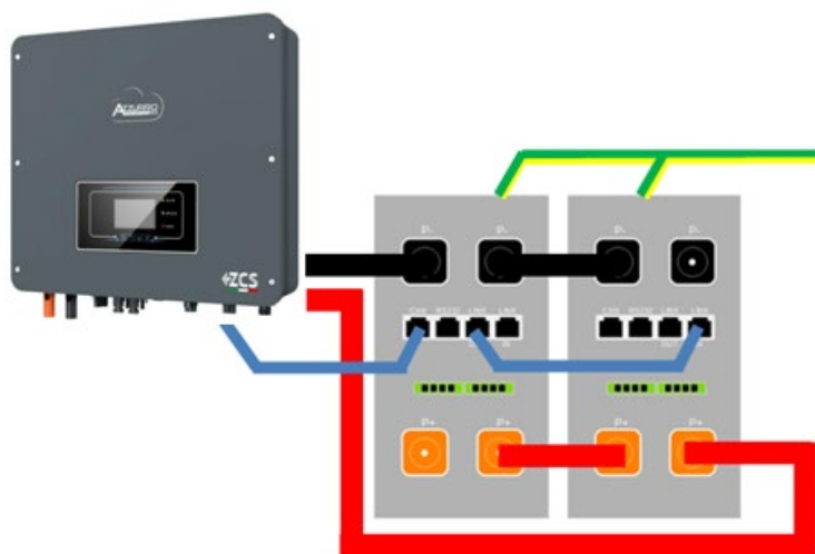
Figura 77 - Collegamento in parallelo di due batterie AZZURRO 5000 PRO
