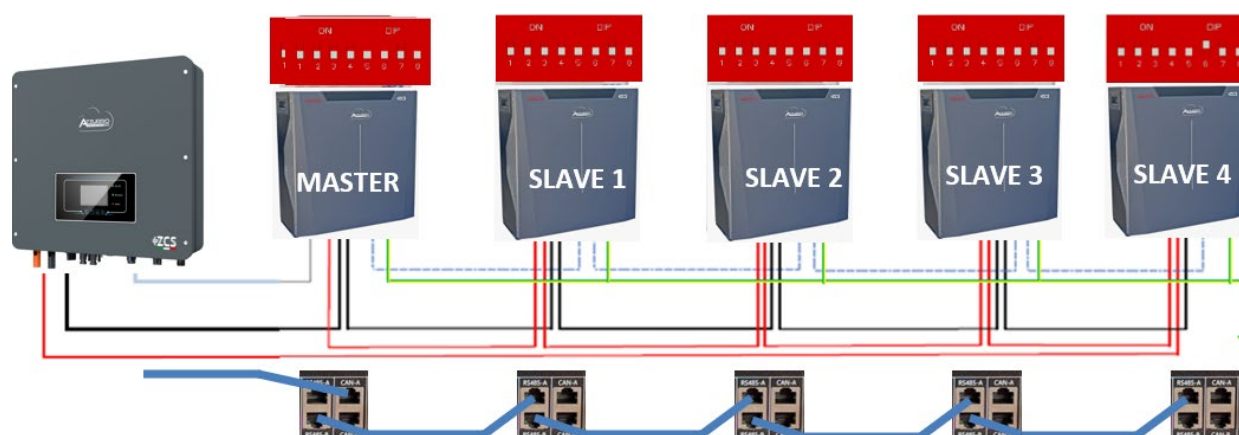
Figura 59 – Collegamento in parallelo di cinque batterie WeCo 5K3XP
