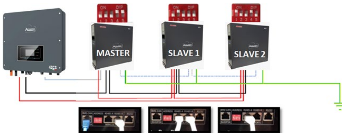
Figura 26 – Collegamento in parallelo di tre batterie WeCo 4k4
