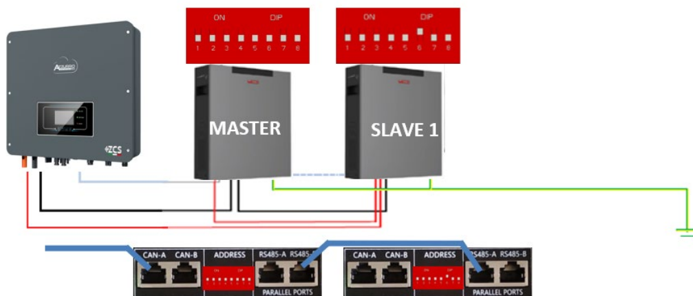
Figura 41 – Collegamento in parallelo di due batterie WeCo 4k4-LT
