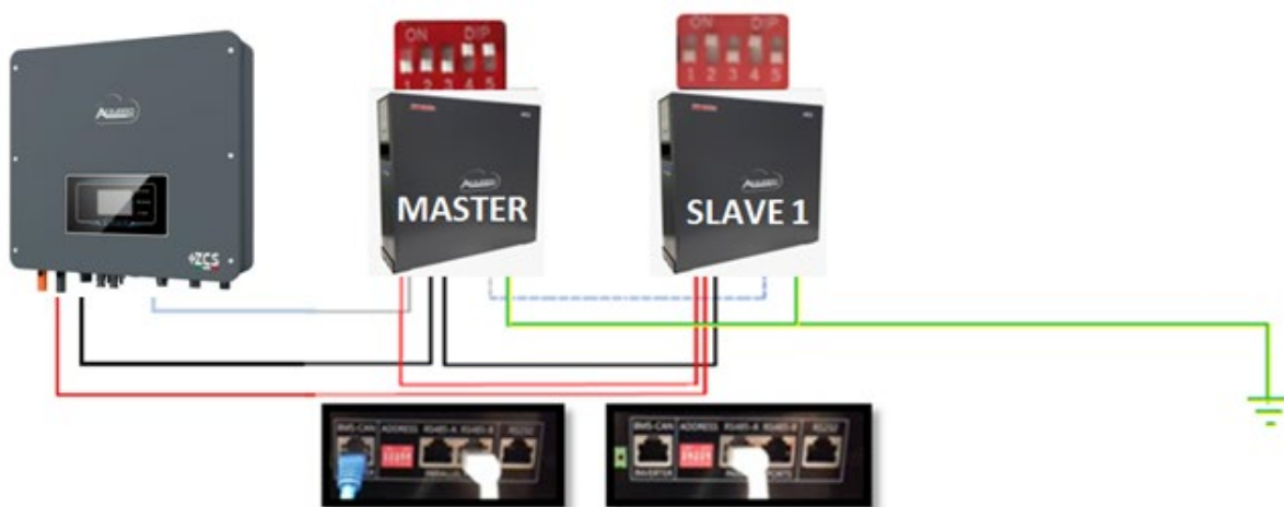
Figura 25 – Collegamento in parallelo di due batterie WeCo 4k4
