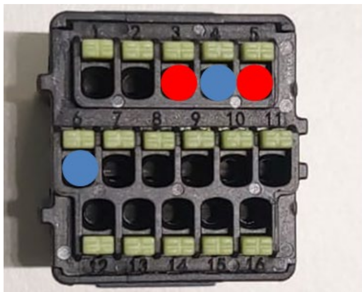
Figura 148 – Collegamento della linea seriale tramite connettore di comunicazione per 3PH HYD5000-HYD20000-ZSS
