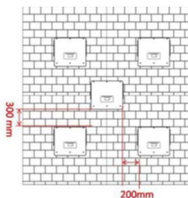
Figura 3 – Posizione di installazione dell'inverter 1PH HYD3000-HYD6000-ZSS-HP
