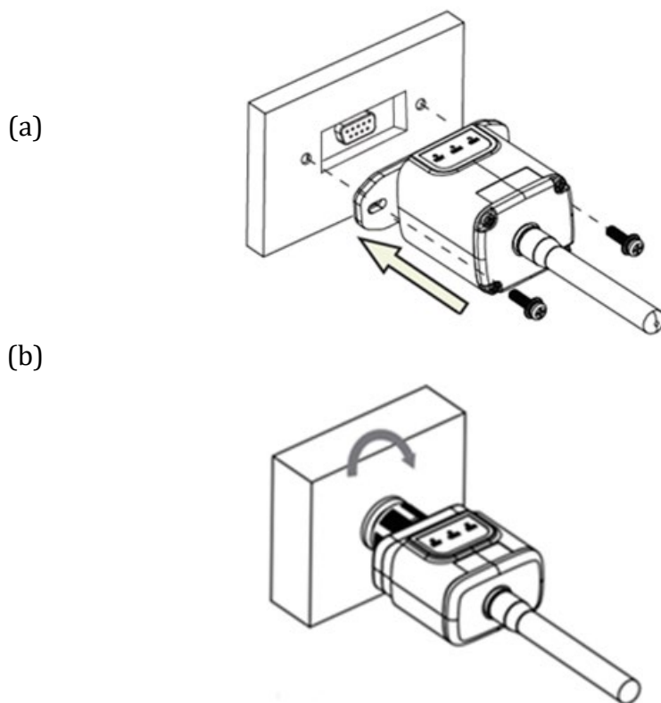
Figura 136 – Inserimento e fissaggio della scheda 4G
