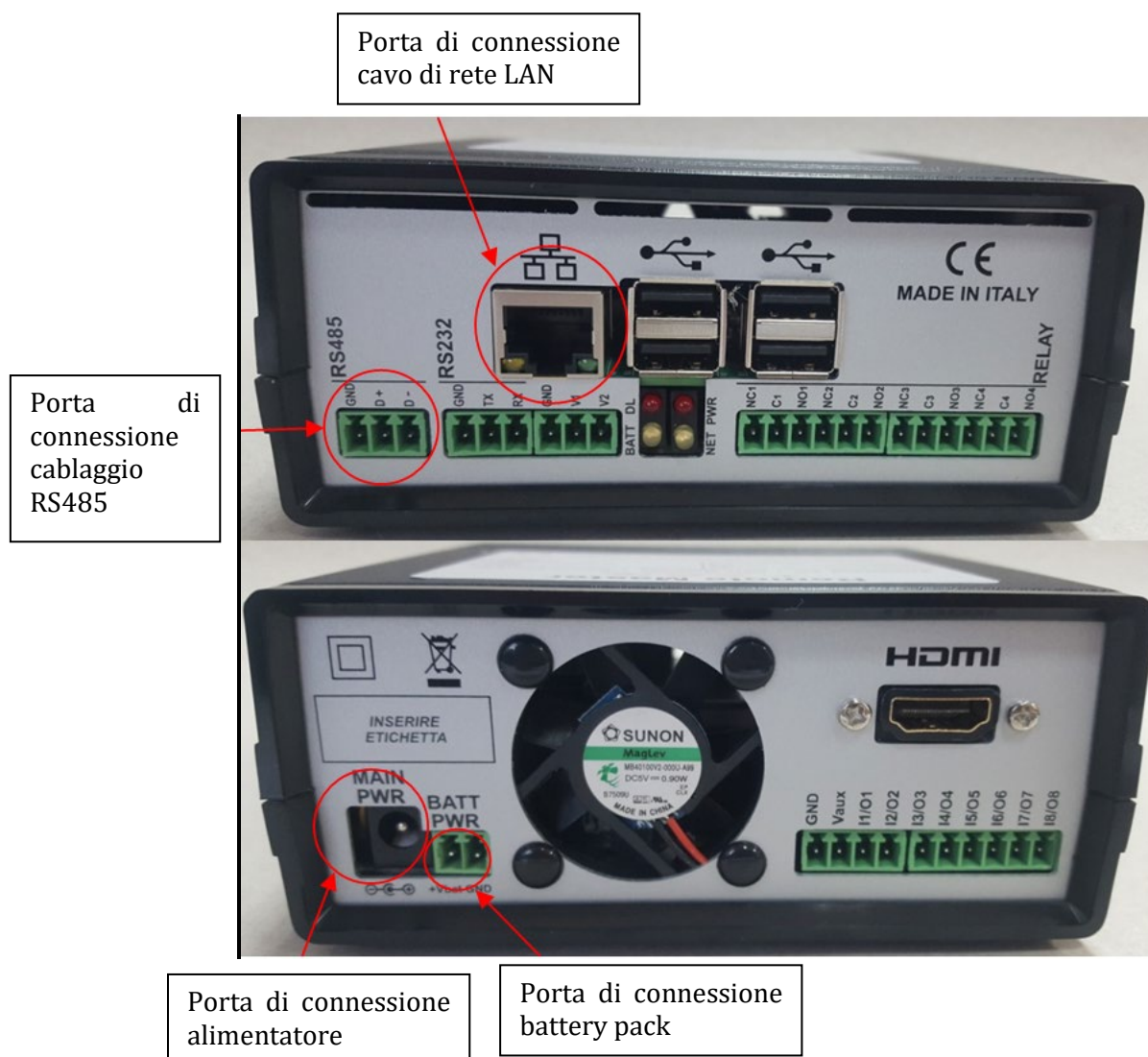
Figura 168: Back Datalogger
