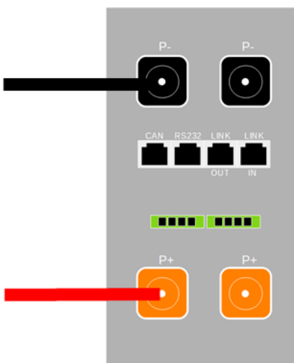
Figura 74 – Morsettiera della batteria AZZURRO 5000 PRO
