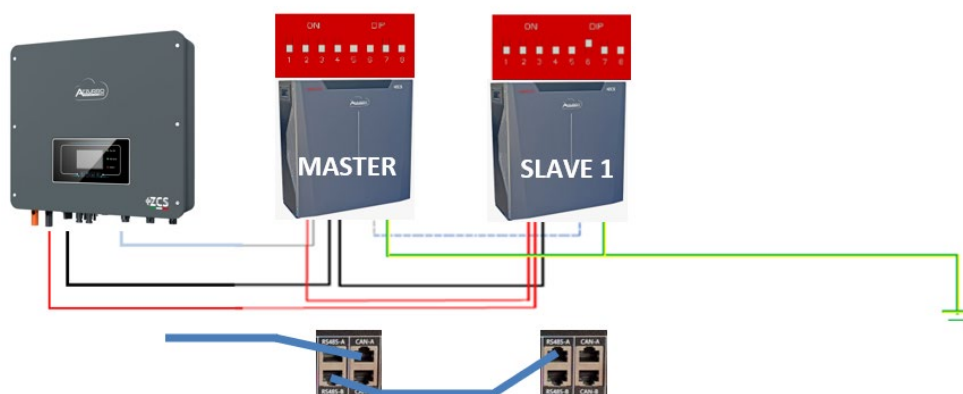
Figura 56 – Collegamento in parallelo di due batterie WeCo 5K3XP
