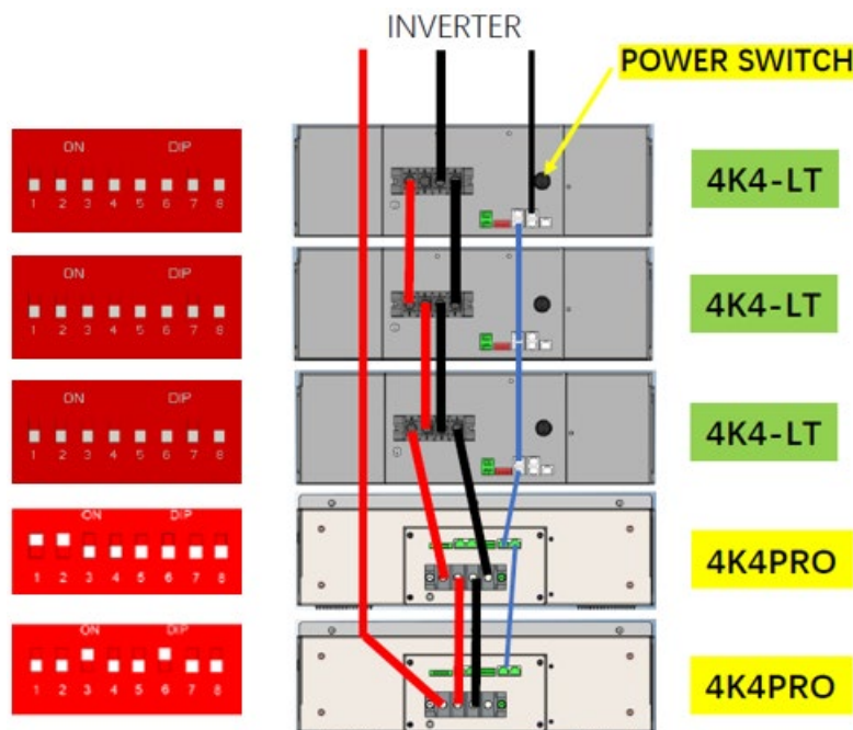
Figura 45 – Collegamento in BATTERIE Weco 4k4-LT e 4k4 PRO
