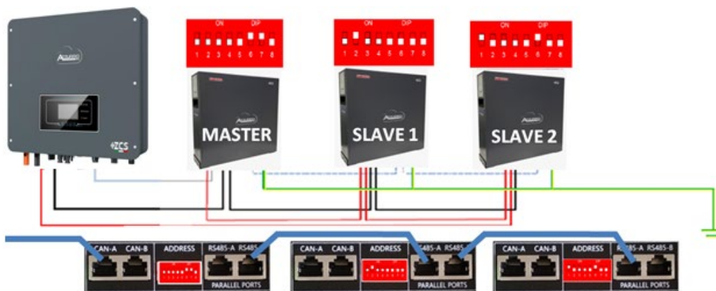
Figura 34 – Collegamento in parallelo di tre batterie WeCo 4k4 PRO
