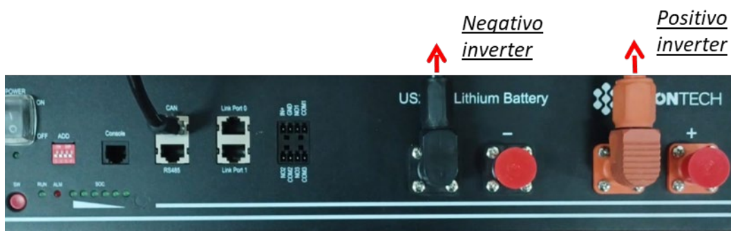
Figura 13- Collegamento del cavo di potenza dalla batteria Pylontech all'inverter
