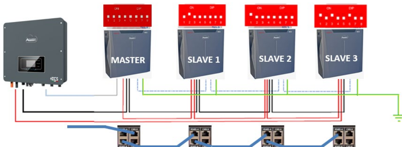
Figura 62 – Collegamento in parallelo con 5K3XP Master e 5K3 Slave
