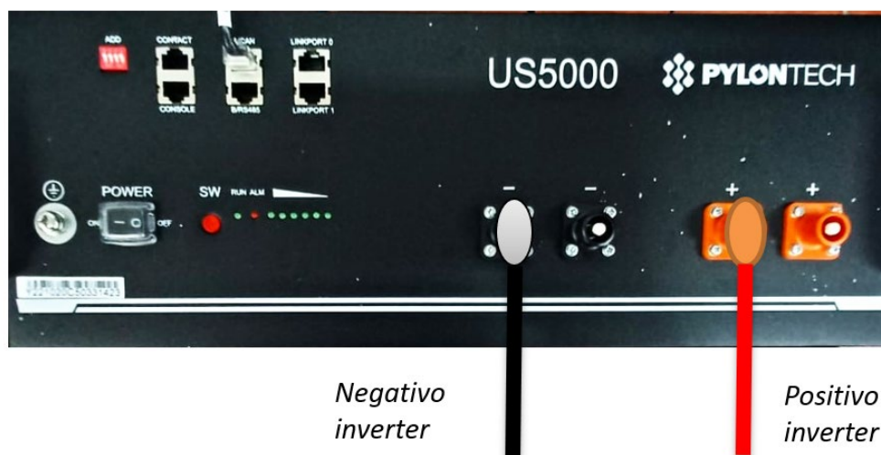
Figura 18- Collegamento del cavo di potenza dalla batteria Pylontech all'inverter
