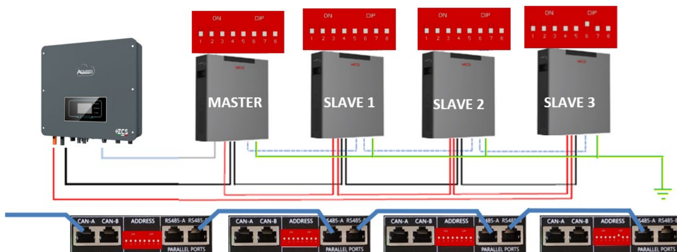
Figura 43 – Collegamento in parallelo di quattro batterie WeCo 4k4-LT
