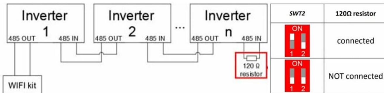
Figura 149 – Posizione dei dip switch per collegare la resistenza di isolamento
