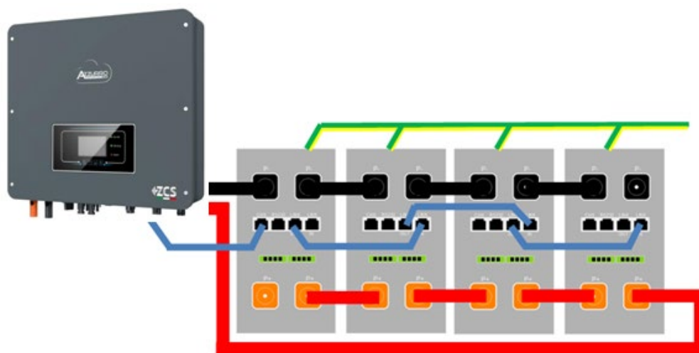
Figura 71 – Collegamento in parallelo di quattro batterie AZZURRO 5000
