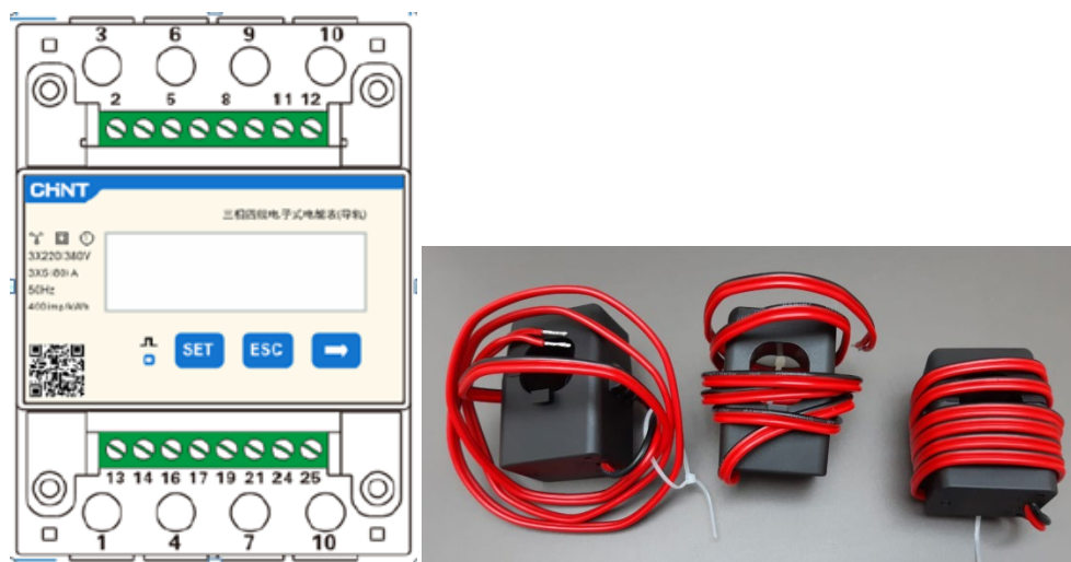
Figura 90 - Meter (a sinistra), sensori CT (a destra)
