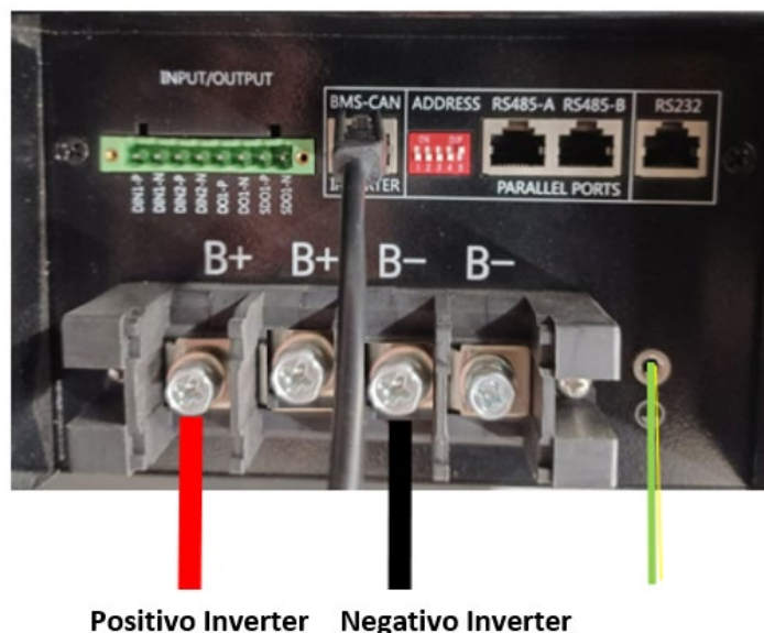
Figura 23- Collegamento del cavo di potenza dalla batteria Weco all'inverter
