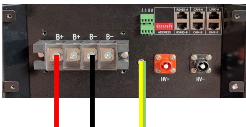
Figura 47 - Collegamento della batteria WeCo 5k3
