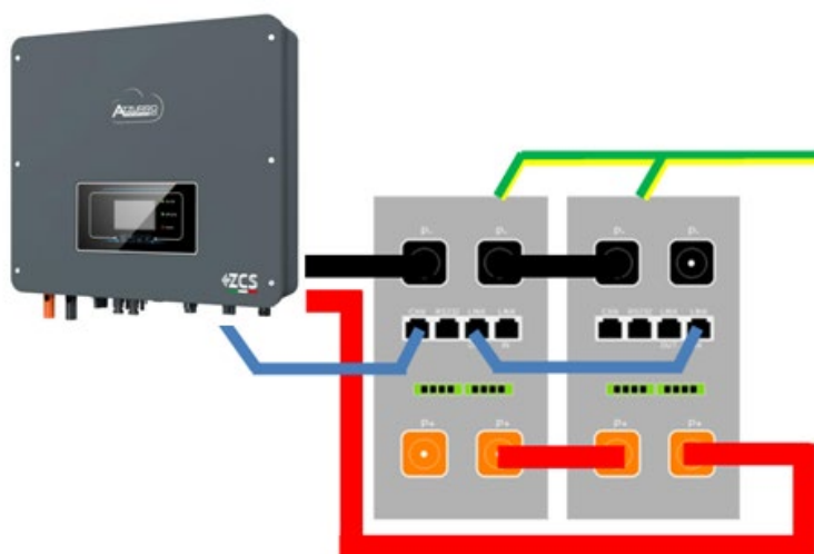
Figura 69 – Collegamento in parallelo di due batterie AZZURRO 5000
