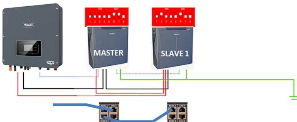
Figura 49 – Collegamento in parallelo di due batterie WeCo 5k3
