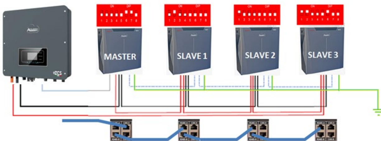
Figura 51 – Collegamento in parallelo di quattro batterie WeCo 5k3
