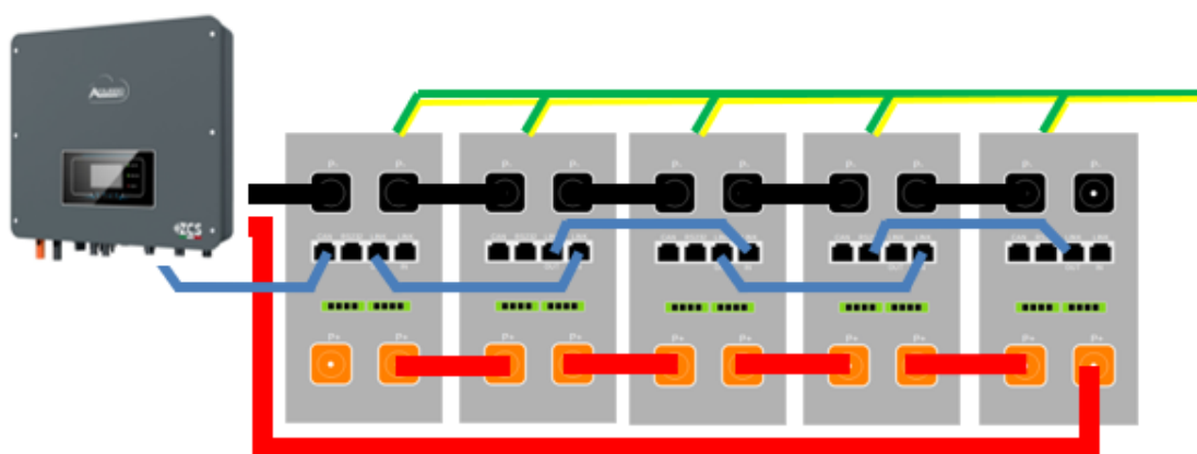
Figura 88 – Collegamento in parallelo di cinque batterie AZZURRO ZSX 5120
