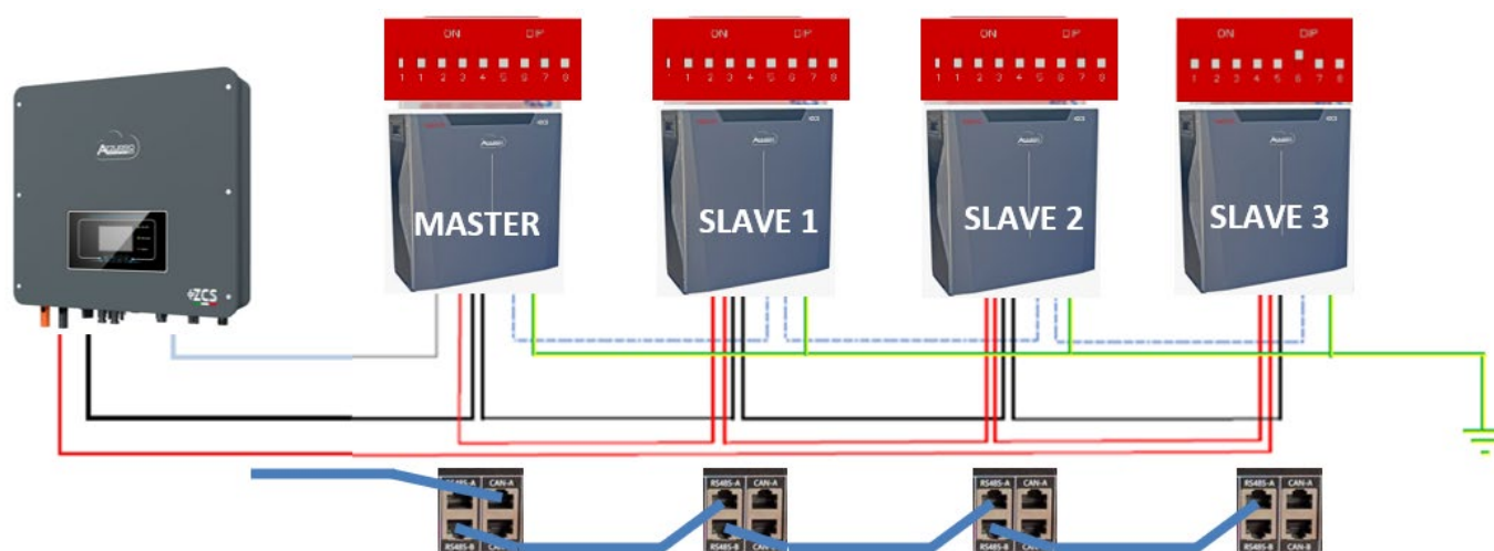
Figura 58 – Collegamento in parallelo di quattro batterie WeCo 5K3XP
