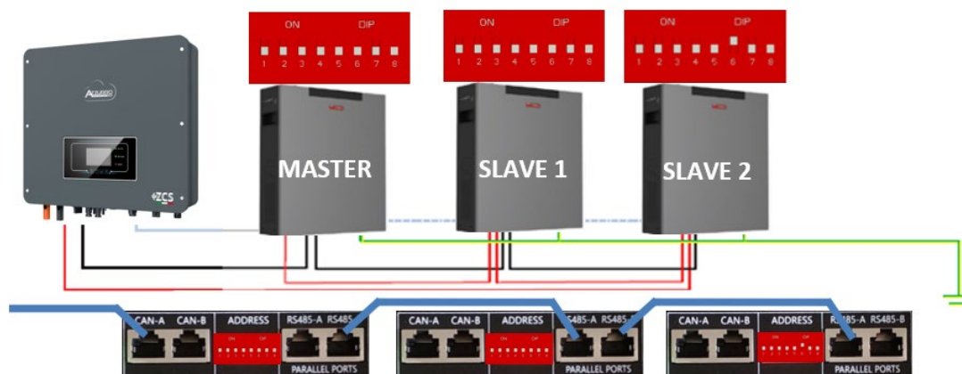
Figura 42 – Collegamento in parallelo di tre batterie WeCo 4k4-LT
