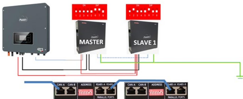
Figura 33 – Collegamento in parallelo di due batterie WeCo 4k4 PRO
