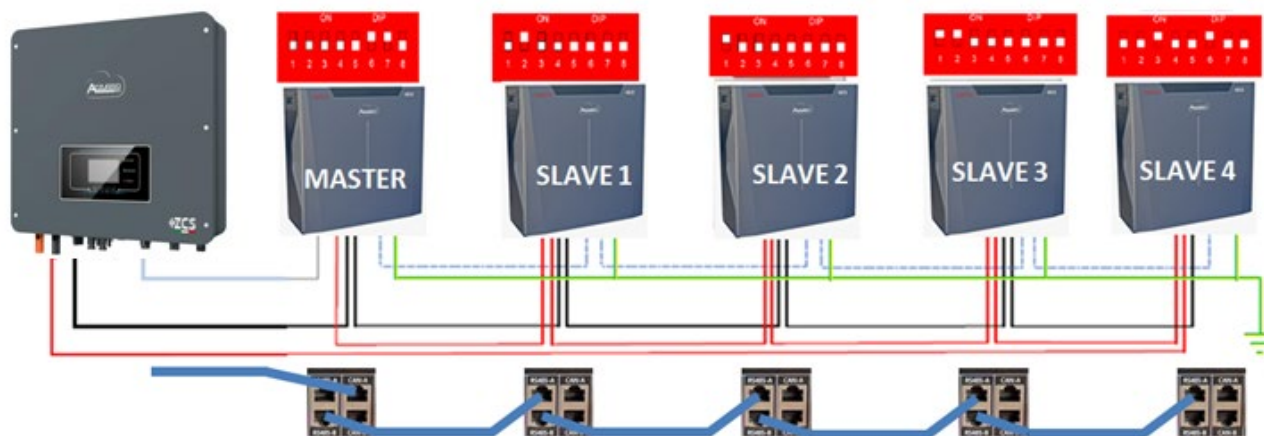
Figura 52 – Collegamento in parallelo di cinque batterie WeCo 5k3
