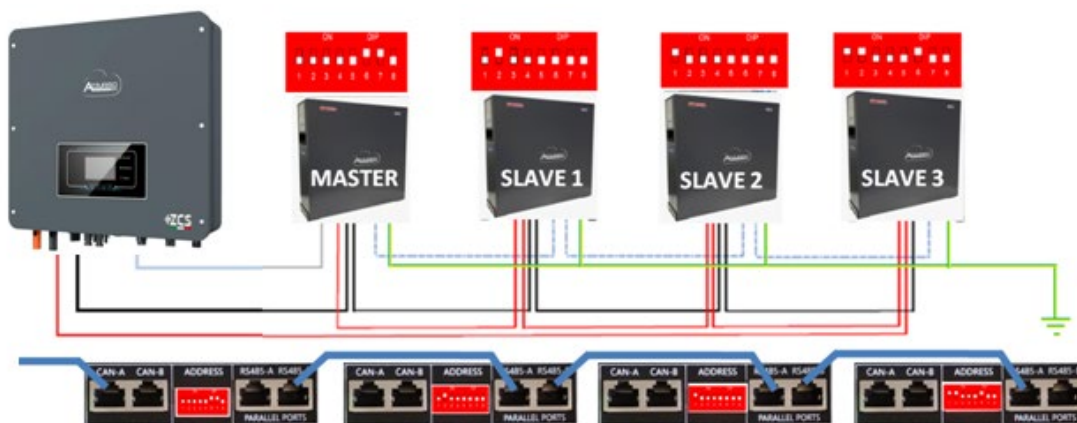
Figura 35 - Collegamento in parallelo di quattro batterie WeCo 4k4 PRO
