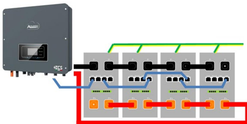
Figura 79 – Collegamento in parallelo di quattro batterie AZZURRO 5000 PRO
