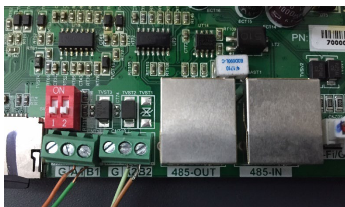
Figura 145 – Collegamento linea seriale tramite morsettiera RS485 e tramite plug RJ45
