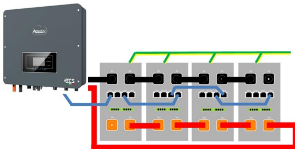
Figura 87 – Collegamento in parallelo di quattro batterie AZZURRO ZSX 5120
