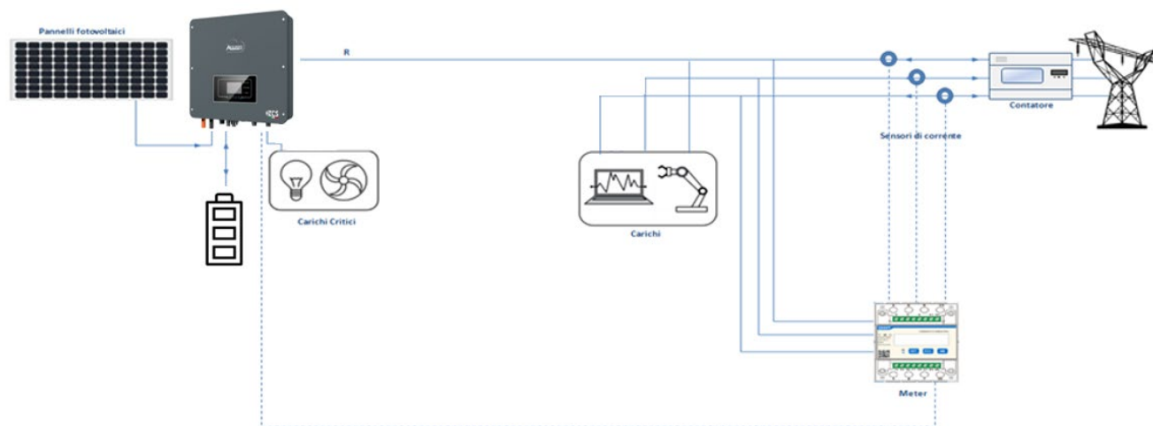
Figura 89 - Schema installazione Ibrido con Meter sullo scambio
