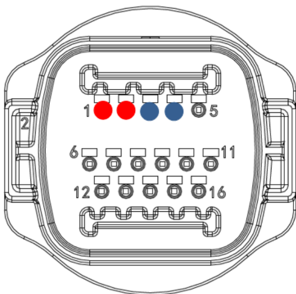
Figura 147 – Collegamento della linea seriale tramite connettore di comunicazione per 1PH 3000-6000 TLM-V3
