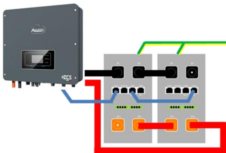
Figura 85 – Collegamento in parallelo di due batterie AZZURRO ZSX 5120
