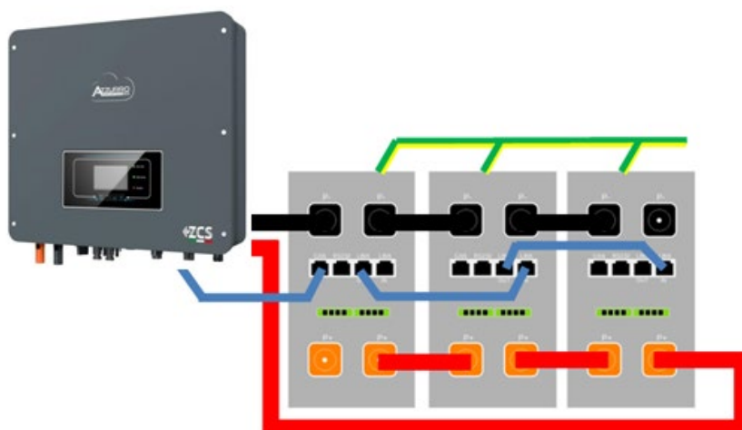
Figura 86 – Collegamento in parallelo di tre batterie AZZURRO ZSX 5120
