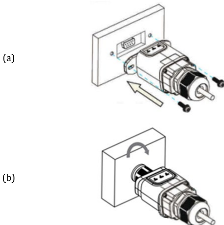
Figura 129 – Inserimento e fissaggio della scheda ethernet
