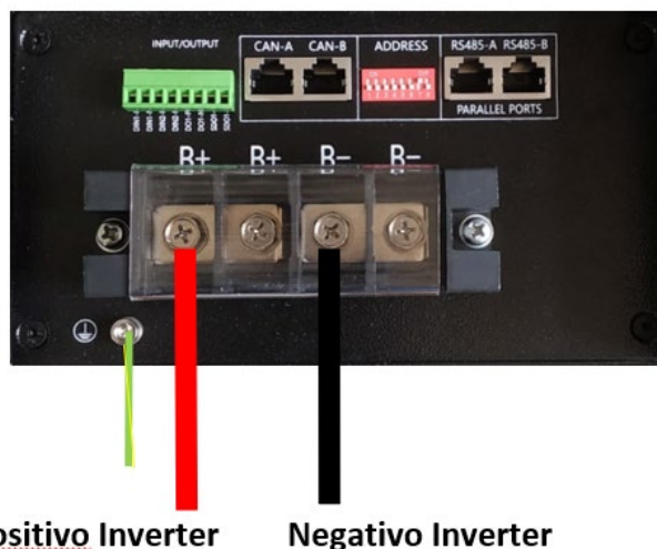
Figura 39- Collegamento del cavo di potenza dalla batteria Weco 4k4-LT all'inverter
