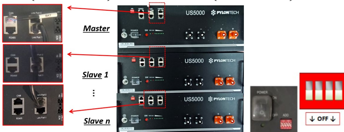
Figura 19 - Collegamento del cavo di comunicazione tra tre batterie Pylontech
