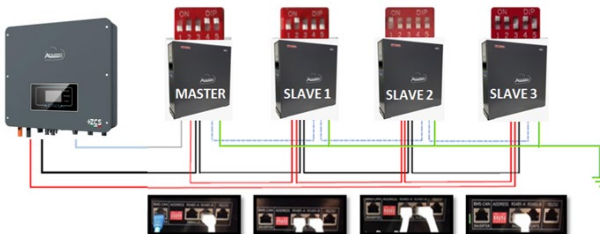
Figura 27 – Collegamento in parallelo di quattro batterie WeCo 4k4
