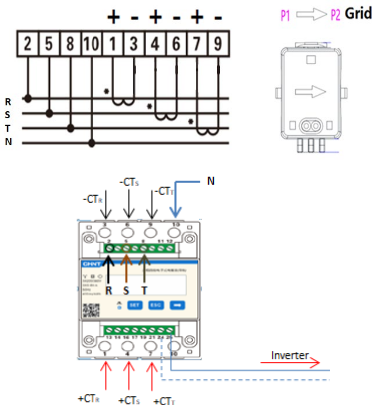
Figura 91 - Collegamenti Meter e sensori
