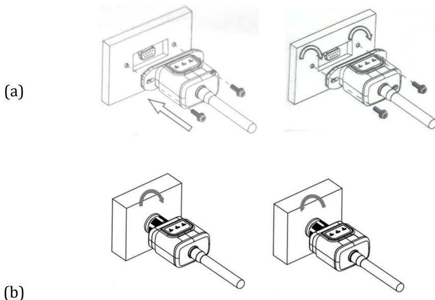
Figura 104 – Inserimento e fissaggio della scheda wifi esterna
