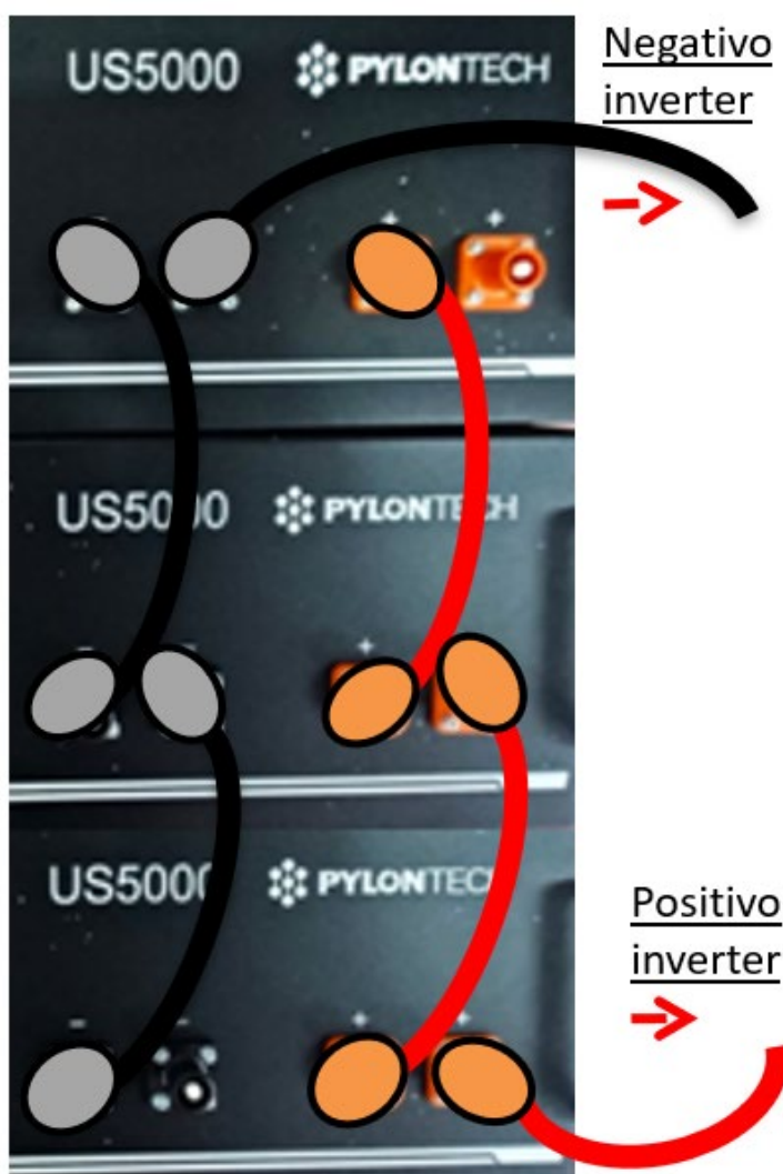
Figura 20 - Collegamento di tre batterie Pylontech in parallelo
