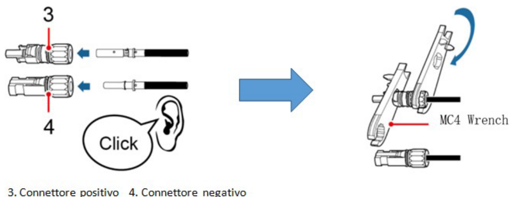
Figura 8 - Preparazione dei connettori fotovoltaici positivo e negativo
