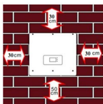
Figura 3 – Posizione di installazione dell'inverter 1PH HYD3000-HYD6000-ZSS-HP
