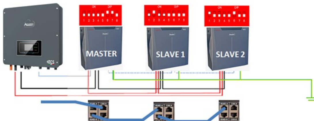
Figura 50 – Collegamento in parallelo di tre batterie WeCo 5k3
