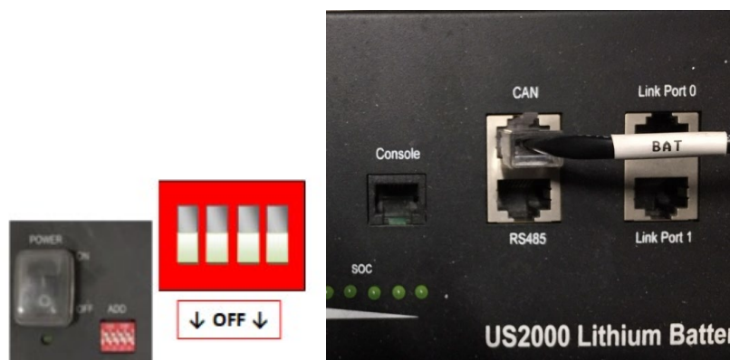
Figura 17- Collegamento del cavo di comunicazione alla batteria Pylontech
