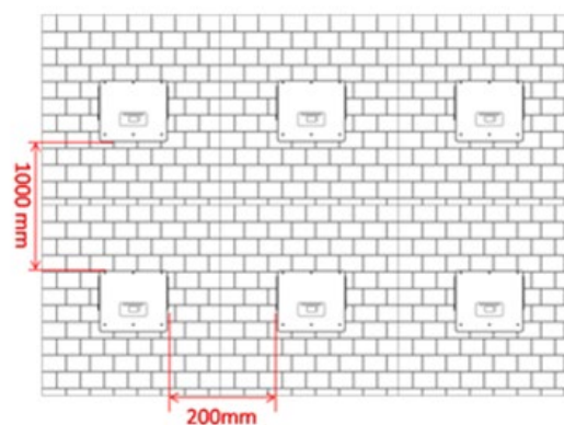
Figura 3 – Posizione di installazione dell'inverter 1PH HYD3000-HYD6000-ZSS-HP
