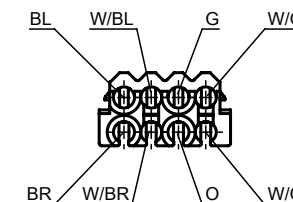
Anschlussbelegung nach TIA/EIA 568-C.2 scale 2:1
