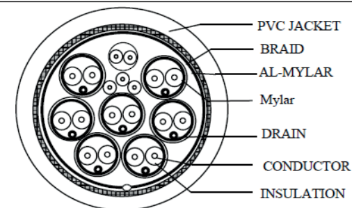
CONSTRUCTION D.W.G
