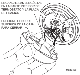
Fig. 9. Montaje del termostato a la placa de fijación.
