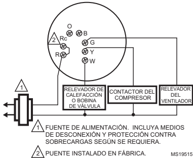
Fig. 4. Conexión típica del termostato T8775C en un sistema de calefacción-enfriamiento con un transformador.
