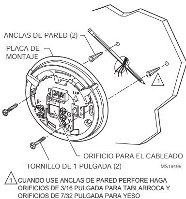
Fig. 1. Cómo montar la placa de fijación al muro.
