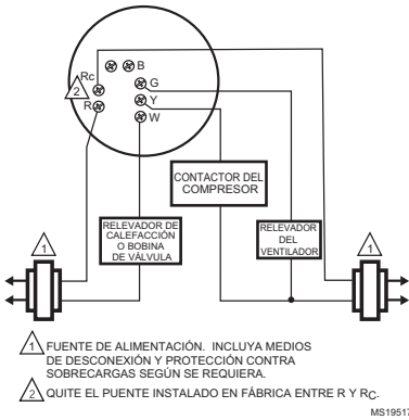
Fig. 5. Conexión típica del termostato T8775C en un sistema de calefacción-enfriamiento con dos transformadores.
