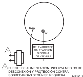
Fig. 2. Conexión típica del termostato T8775A en un sistema exclusivamente de calefacción.
