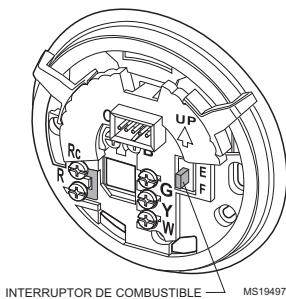
Fig. 7. Interruptor de combustible.
