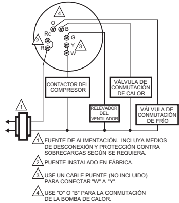
Fig. 6. Conexión típica del termostato T8775C en un sistema de bomba de calefacción de una etapa.
