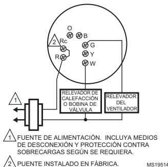
Fig. 3. Conexión típica del termostato T8775C en un sistema exclusivamente de calefacción con ventilador.
