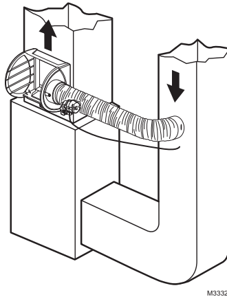
Fig. 12. Instalación de la tubería del interruptor de presión.
