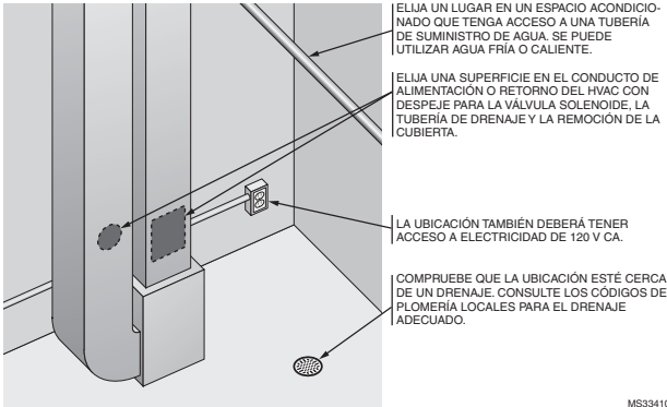
Fig. 2. Ubicaciones de instalación típicas para el humidificador.
