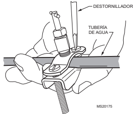
Fig. 8. Instalación de la válvula de asiento.
