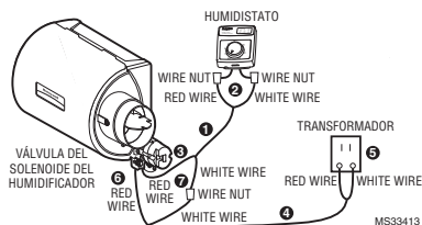
Fig. 16. Cableado de los controles y el HE240.
