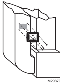
Fig. 15. Fije el soporte de base al conducto.
