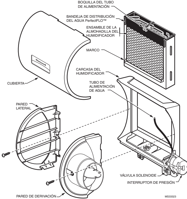
Fig. 4. Desensamblaje del humidificador.
