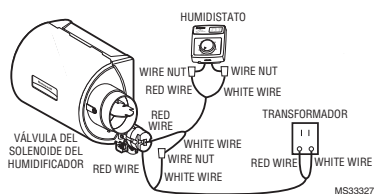
Fig. 17. Cableado de los controles y el HE280.
