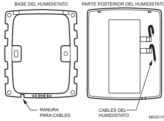
Fig. 13. Base del humidistato y vista posterior.
