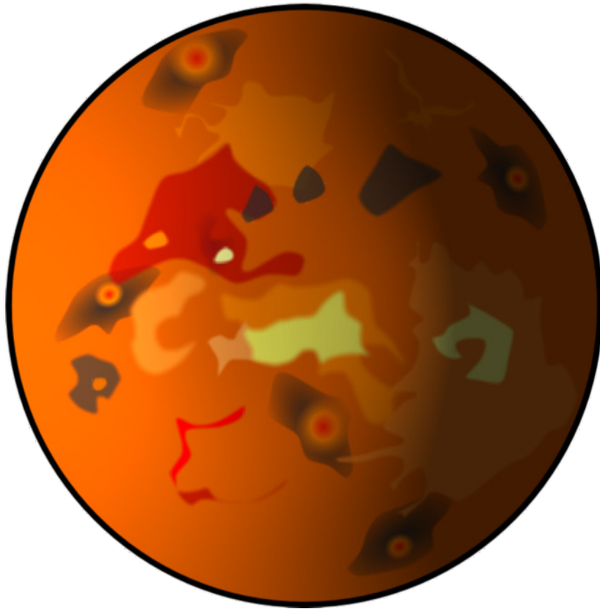
Venus
