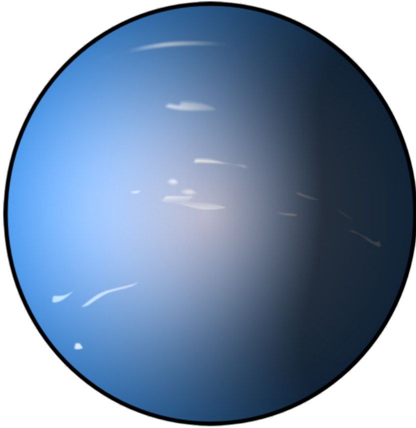
Neptun
