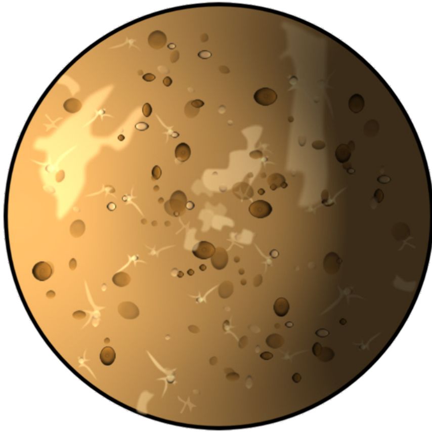
Merkur
