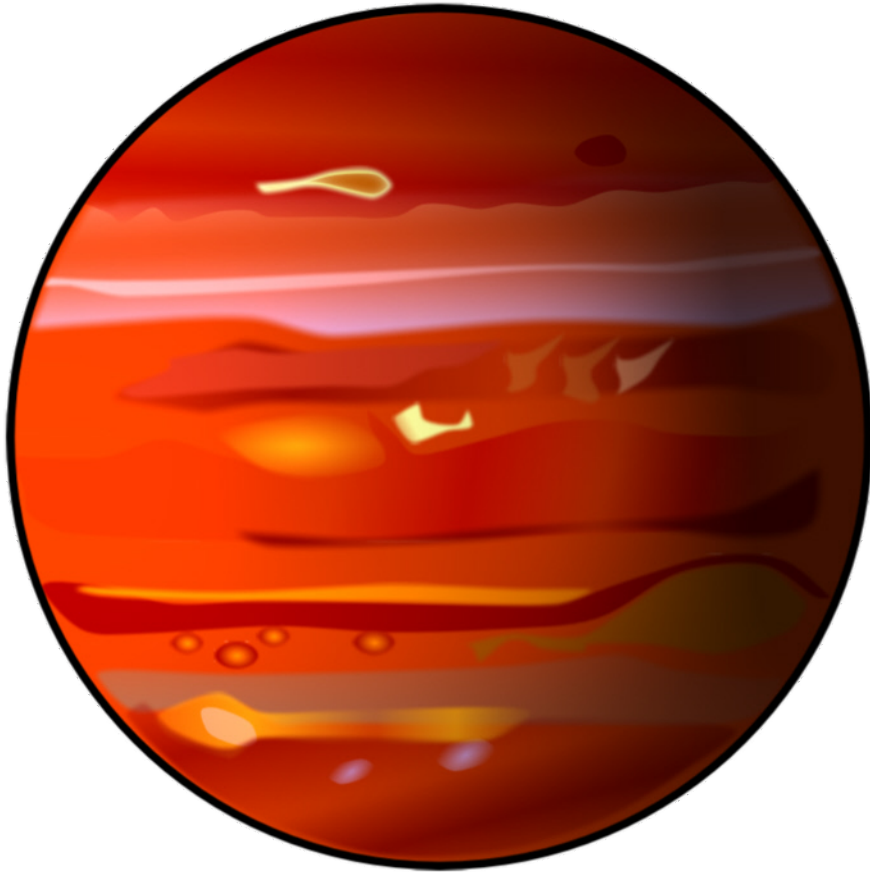
Jupiter
