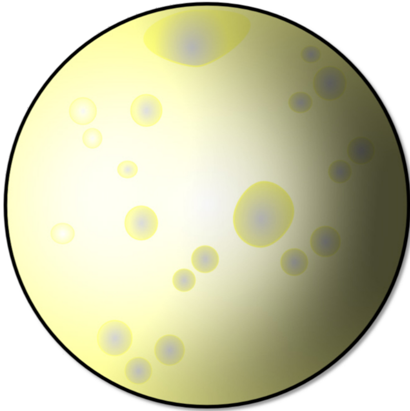
Månen
