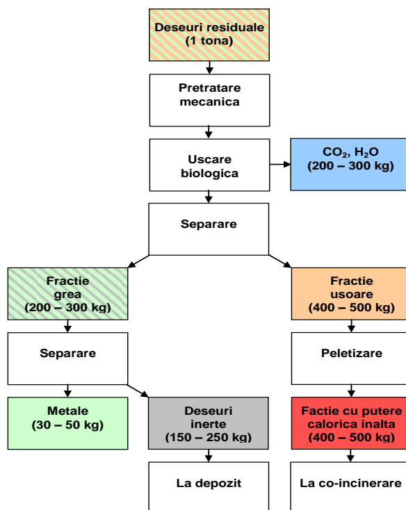
Figura 7-16 TMB cu biouscarea – schema fluxului
