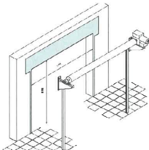
Secțiune tracțiune integrală pe motor lateral
