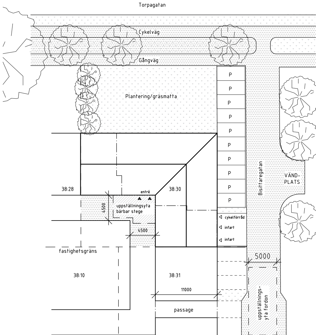
SITUATIONSPLAN SKALA 1:400
