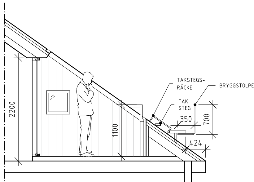
UTSNITT UTRYMNING TERRASS
