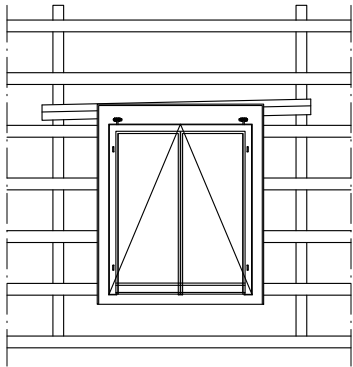
TF1: MONTERINGSPRINCIP
