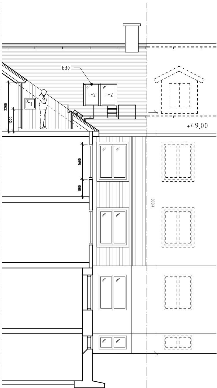
SEKTION B-B
