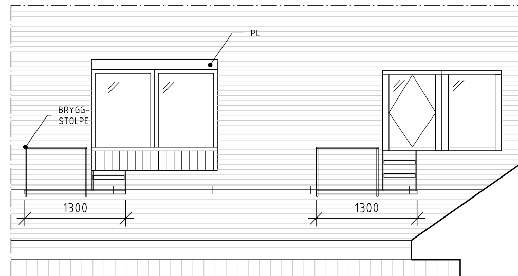
UTSNITT ELEVATION UTRYMNING FÖNSTER OCH TERRASS
