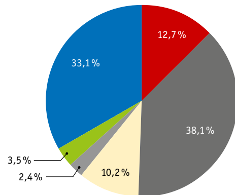
Energieträgermix Deutschland
