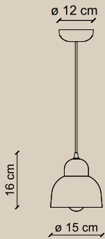
art. C2611 peso netto / net weight Kg 0,86 1 x MAX 53W E27
