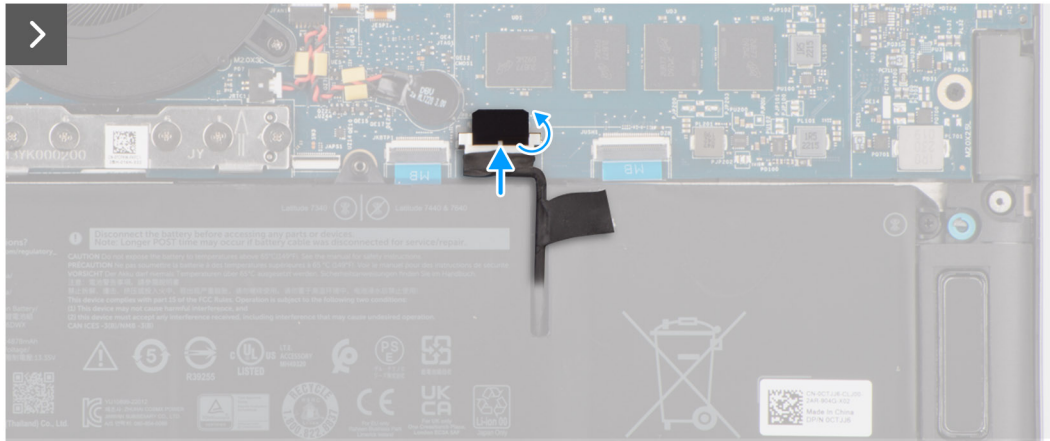
Abbildung 19. Installieren der Bodenabdeckung
