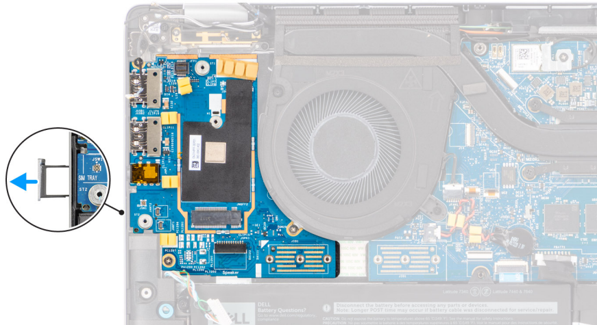
Abbildung 14. Entfernung der I/O-Zusatzplatine
