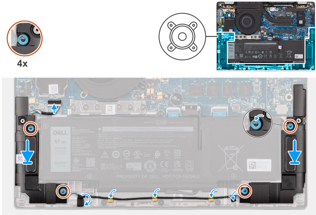
Abbildung 34. Installieren der Lautsprecher (Mainstream)
