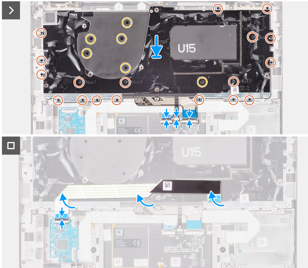
Abbildung 81. Installieren der Tastatur
