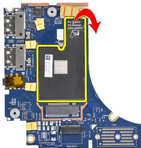
Abbildung 73. Latitude 7450 2-in-1 in der 4G-WWAN-Konfiguration (Dichtungsaufkleber)
