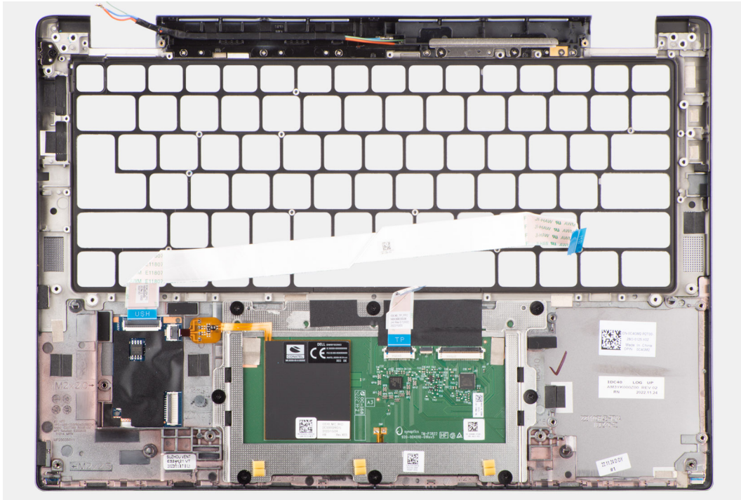
Abbildung 85. Installieren der Handauflagenbaugruppe
