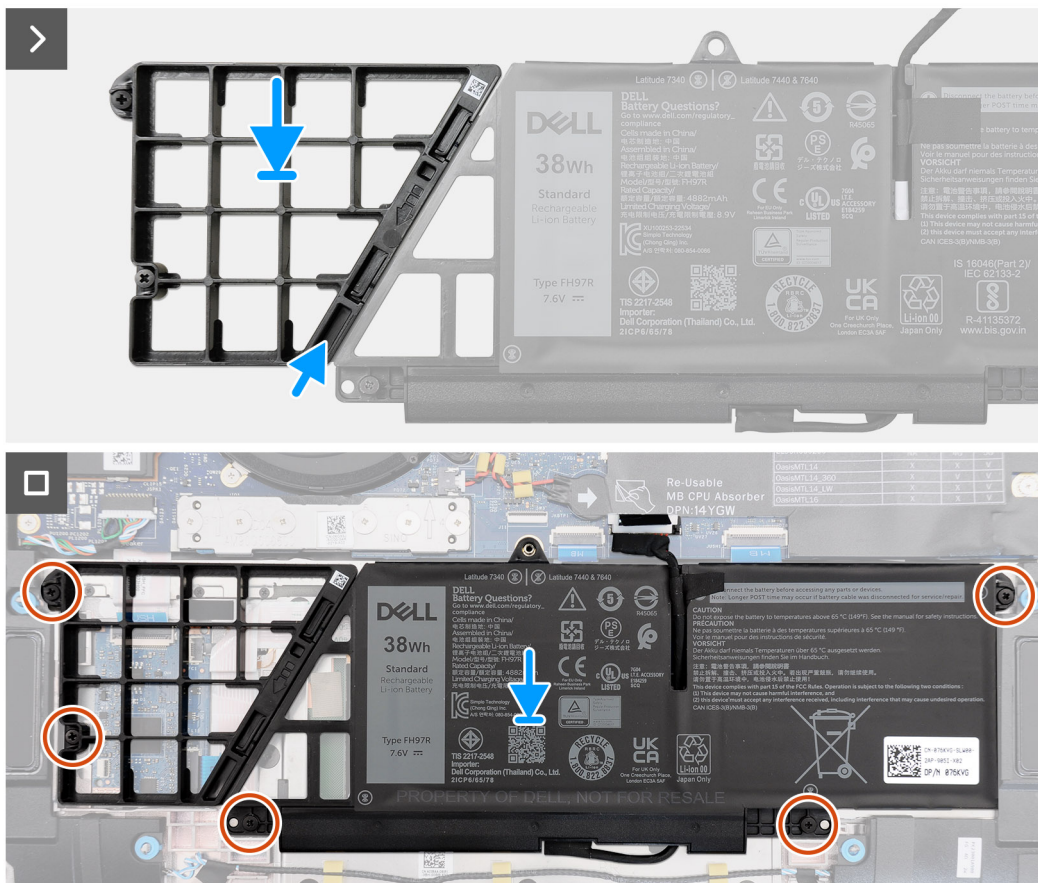
Abbildung 39. Installieren des 2-Zellen-Akkus
