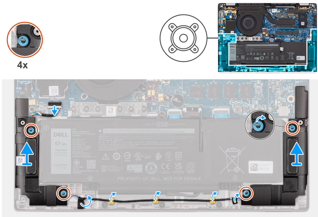
Abbildung 33. Entfernen der Lautsprecher (Mainstream)
