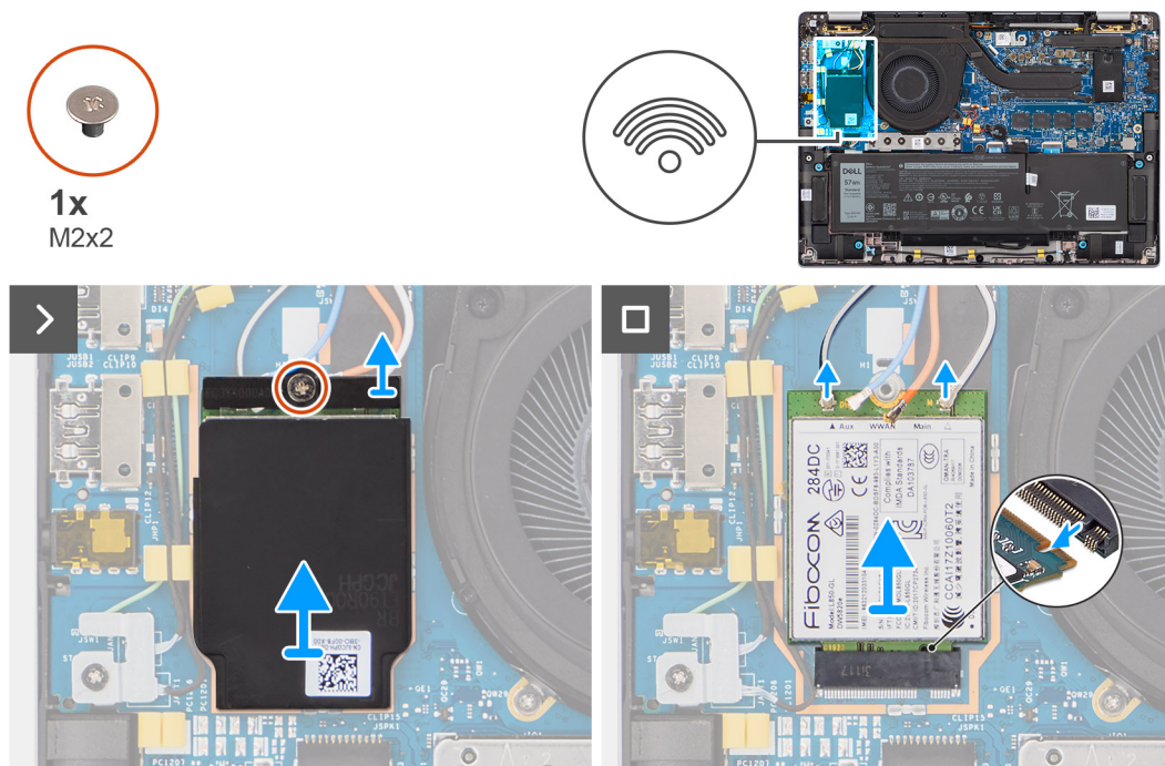
Abbildung 24. Entfernen der 4G-WWAN-Karte
