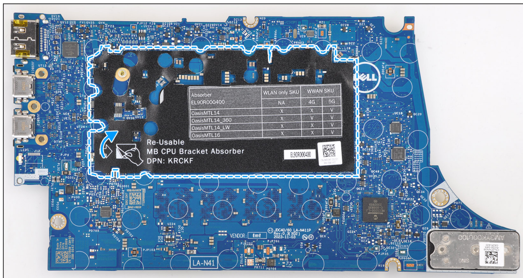
Abbildung 62. Absorber der CPU-Halterung
