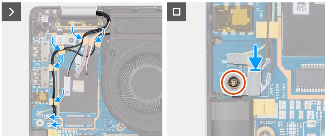
Abbildung 55. Installieren der Displaybaugruppe
