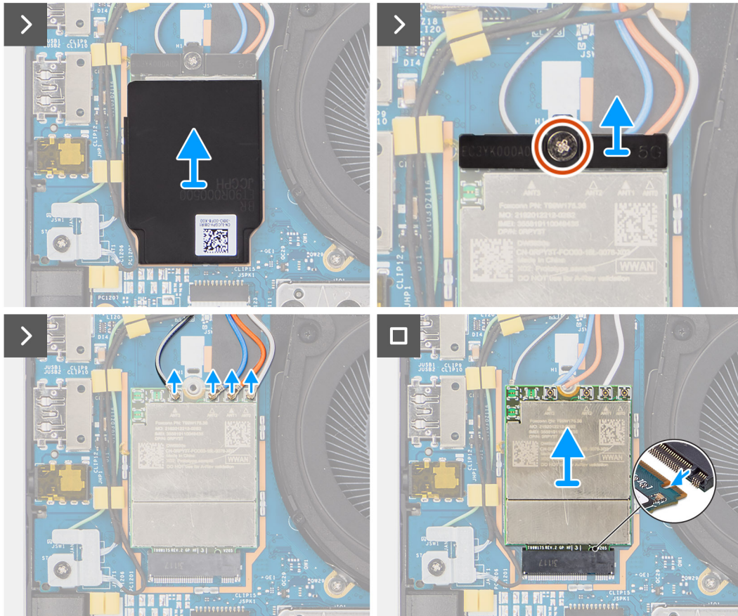
Abbildung 26. Entfernen der 5G-WWAN-Karte
