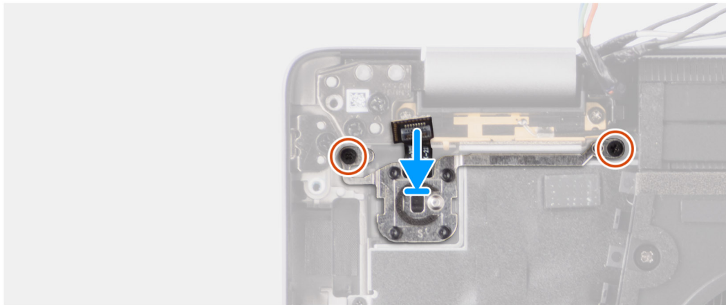
Abbildung 77. Installieren des Netzschalters mit optionalem Fingerabdruck-Lesegerät
