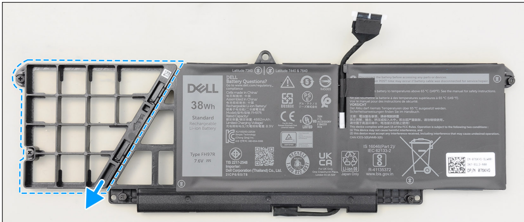
Abbildung 38. Entfernen des 2-Zellen-Akkus
