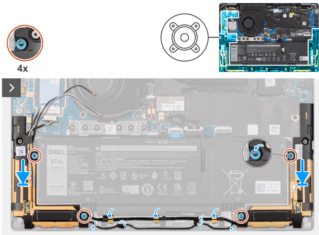
Abbildung 31. Installieren der Lautsprecher (Ultralight)
