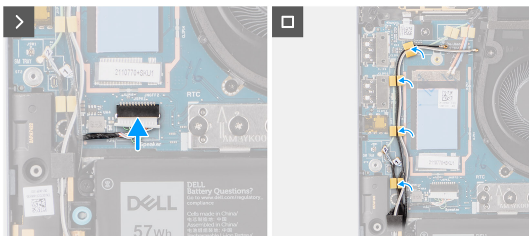
Abbildung 32. Installieren der Lautsprecher (Ultralight)
