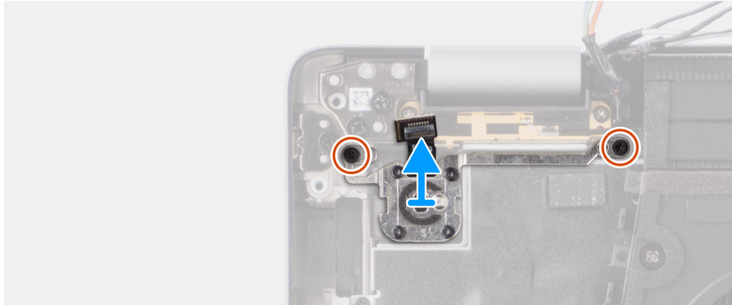
Abbildung 76. Entfernen des Netzschalters mit optionalem Fingerabdruck-Lesegerät
