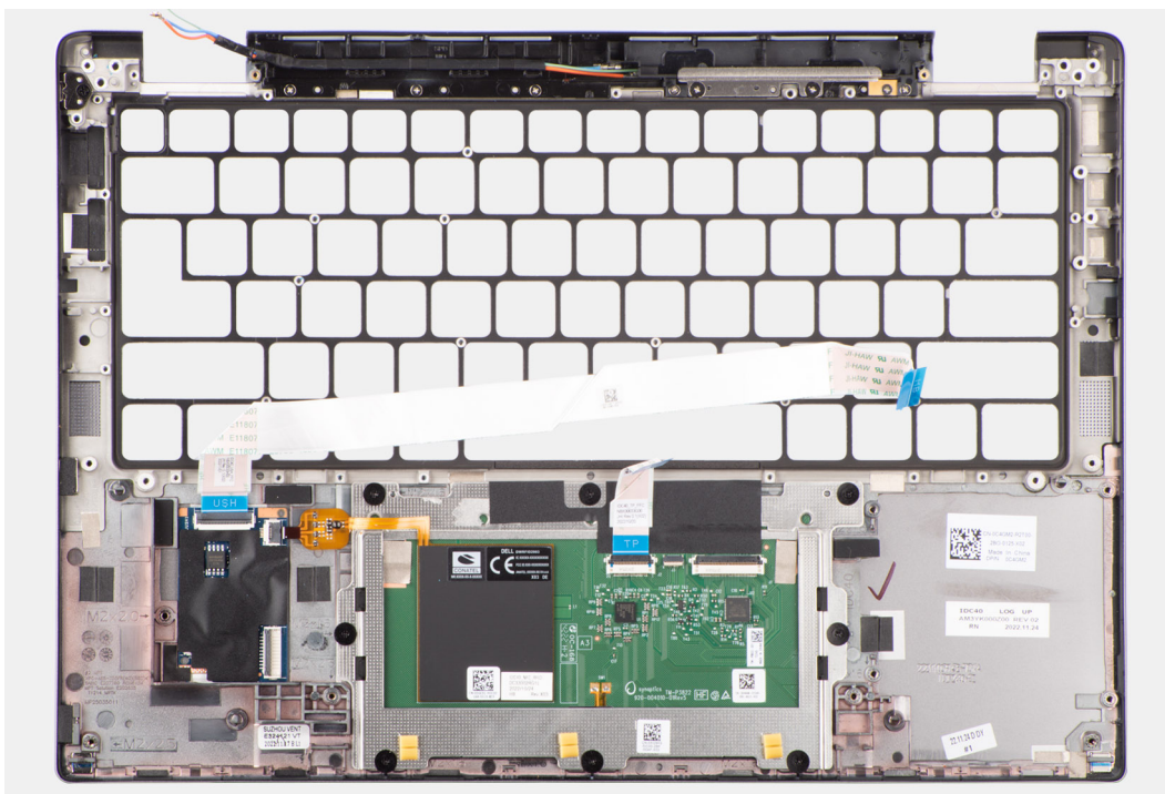
Abbildung 84. Entfernen der Handauflagenbaugruppe
