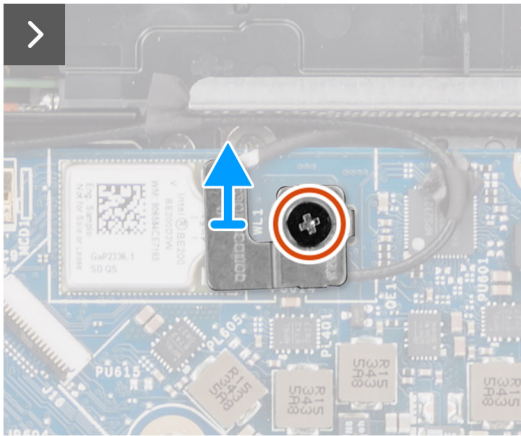
Abbildung 66. Entfernen des WLAN-Antennenmoduls
