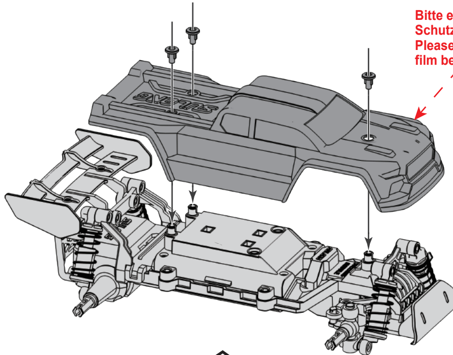
Karosserie / Bodyshell 1x
