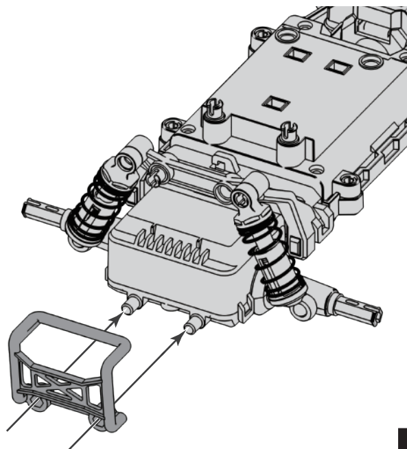
Hinterer Stoßfänger Rear Bumper F2-2 1x
