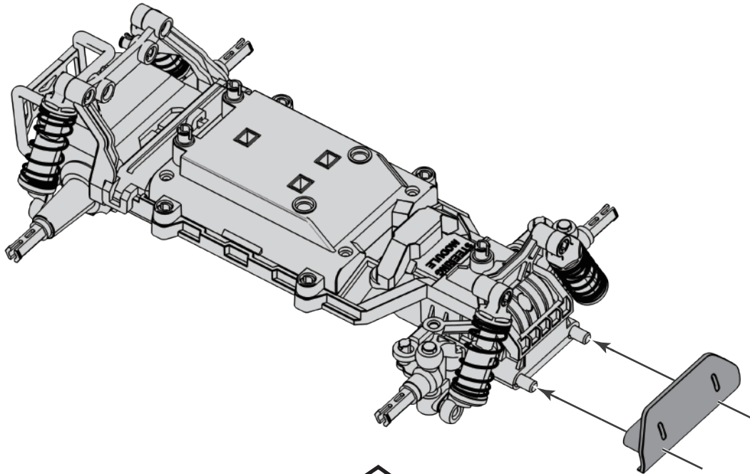
Stoßfänger / Bumper F2-1 1x
