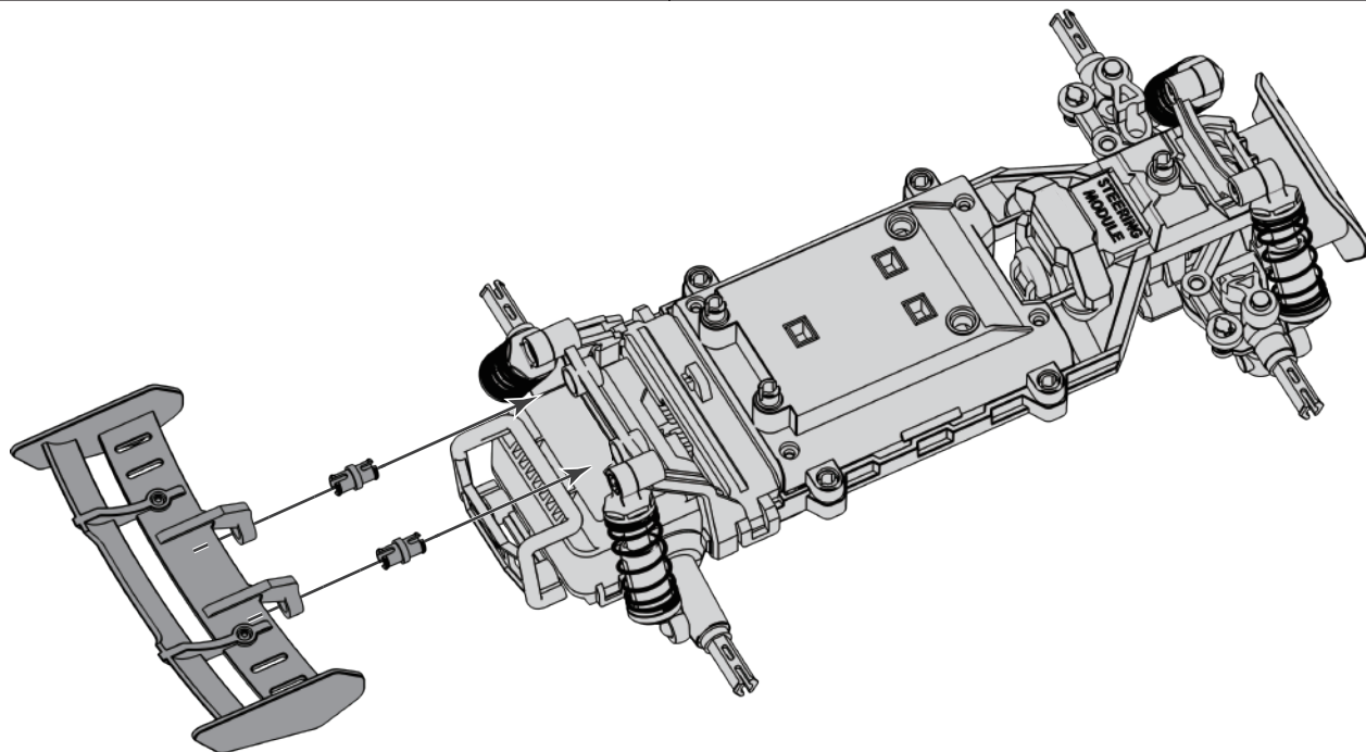
Heckflügel / Tail Fin F2-3 1x
