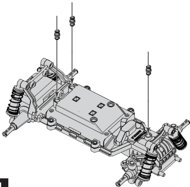
Verbinder / Latch C1 3x
