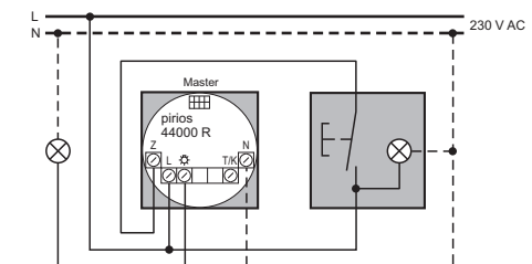
Fig. 2 Tasterfunktion Retrigger
