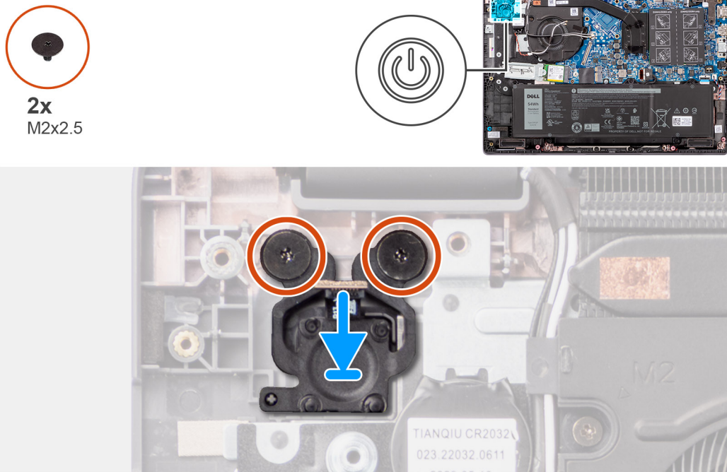
Abbildung 40. Einbauen des Netzschalters
