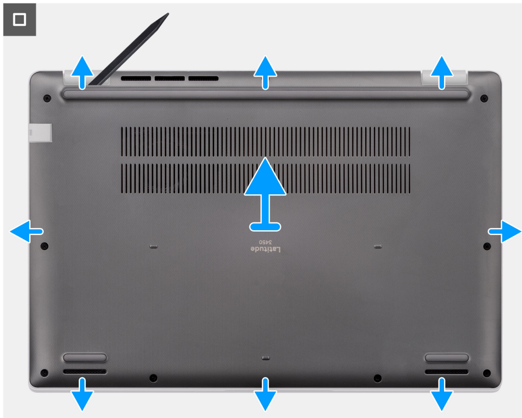
Abbildung 10. Entfernen der Bodenabdeckung
