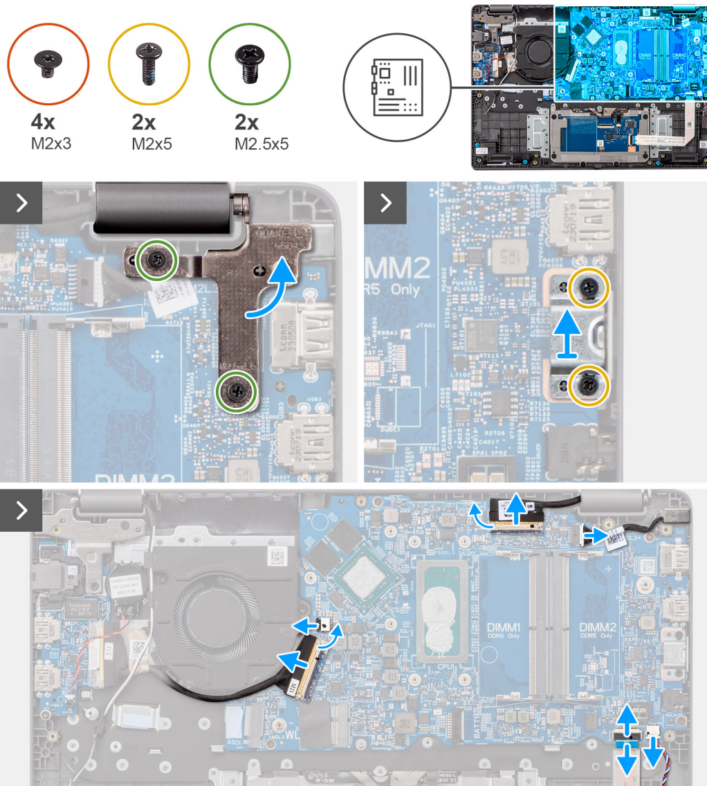
Abbildung 42. Entfernen der Systemplatine
