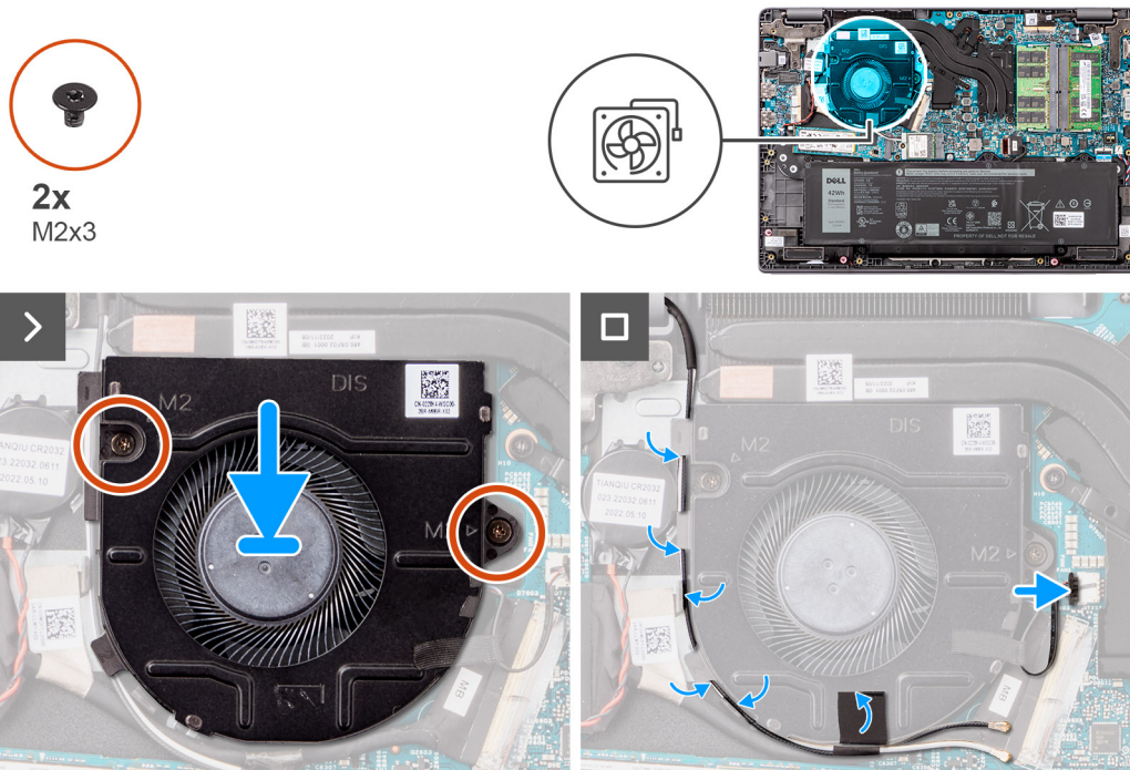
Abbildung 34. Einbauen des Lüfters
