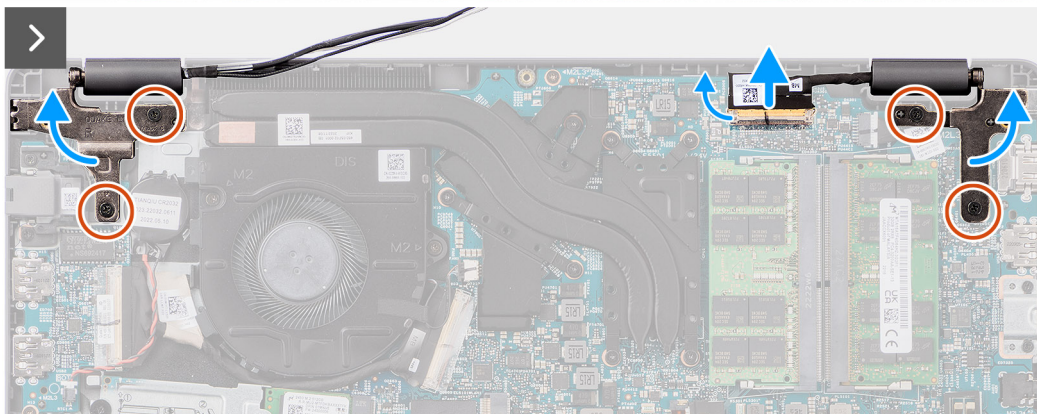
Abbildung 47. Entfernen der Bildschirmbaugruppe
